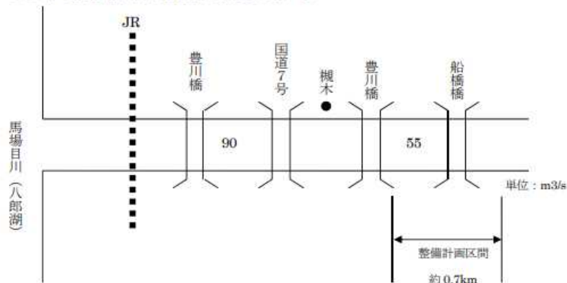
図一12 豊川の流量配分図
