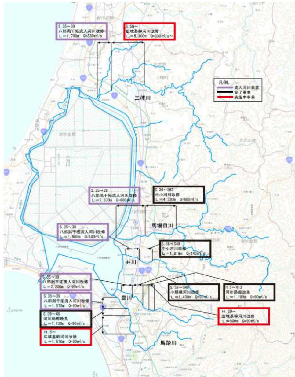
図一2 馬場目圏域の河川改修状況
