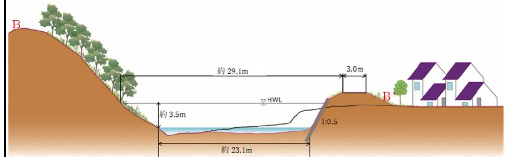
図- 2 3 富津内川横断面図
