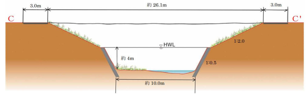
図－2 4 内川川横断面図
