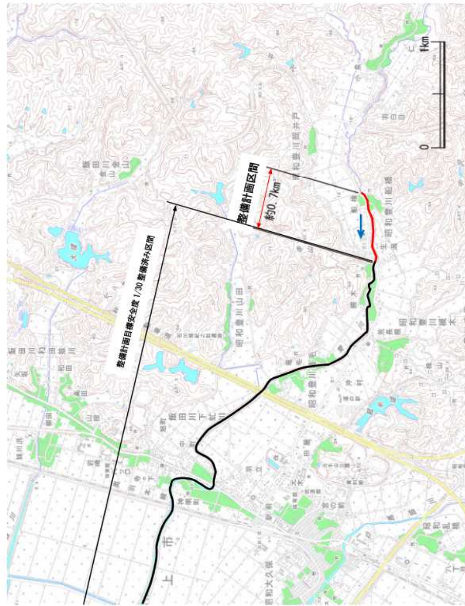
図一13 豊川平面図
