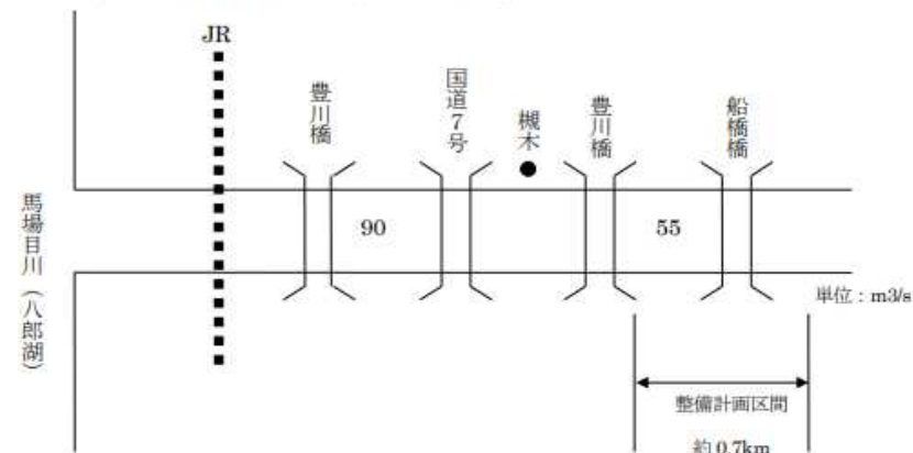
図一12 豊川の流量配分図
