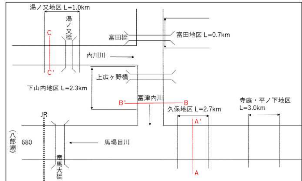
図-20 馬場目川、富津内川、内川川流量配分図
