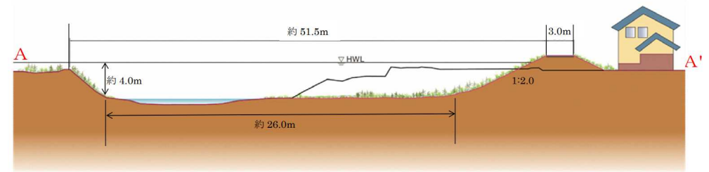
図一 2 2 馬場目川横断面図
