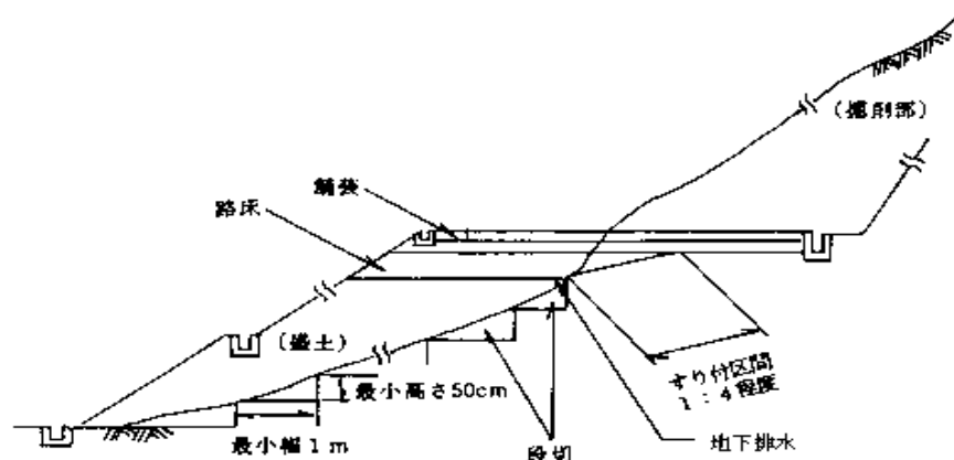
図4-2 盛土基礎地盤の段切
