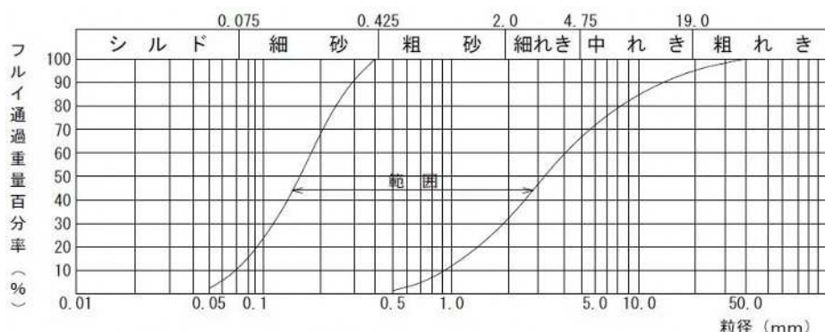
図 5-1 使用砂の粒径加積曲線
