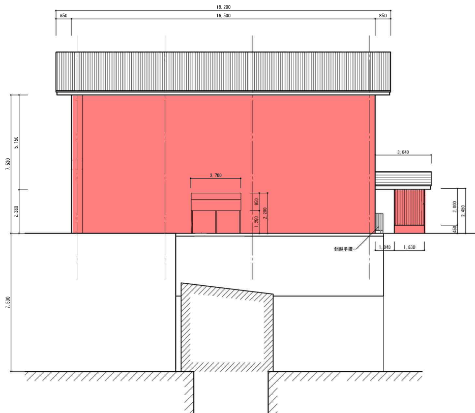
西立面図 S=1:100
