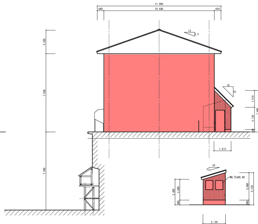
南立面図 S=1:100
