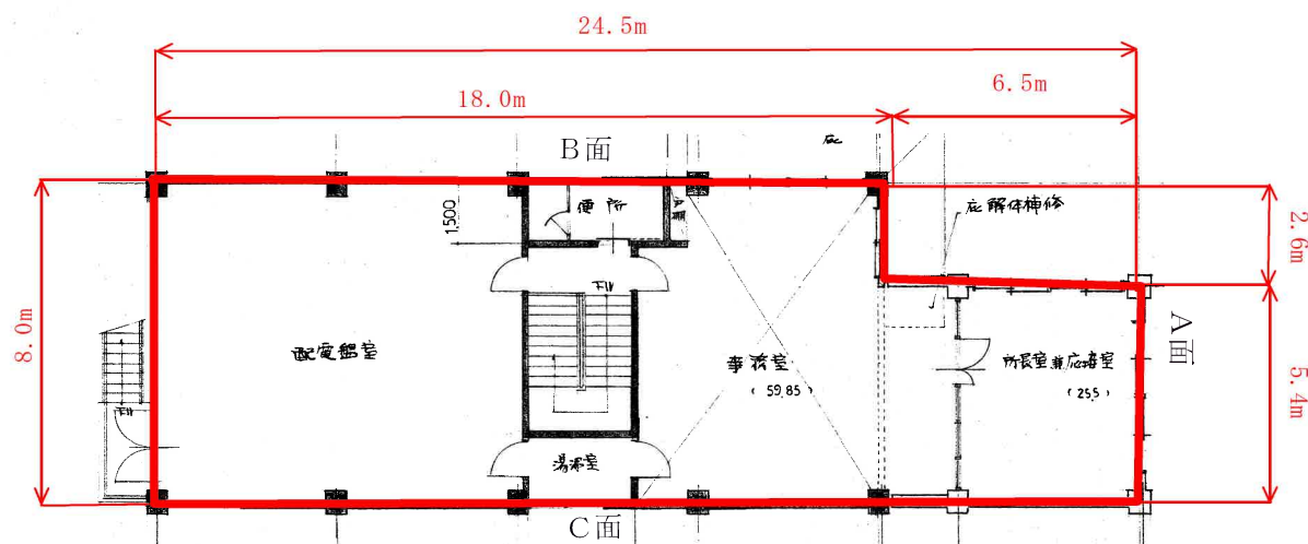
付属建屋 2階平面図
