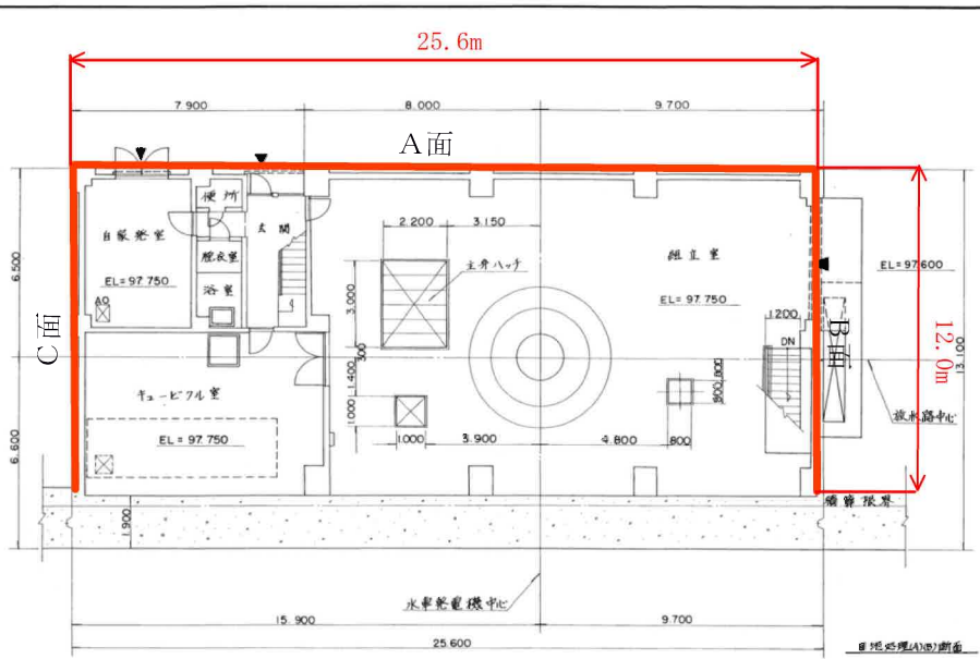
1階平面図
