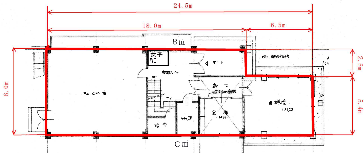
付属建屋 1階平面図
