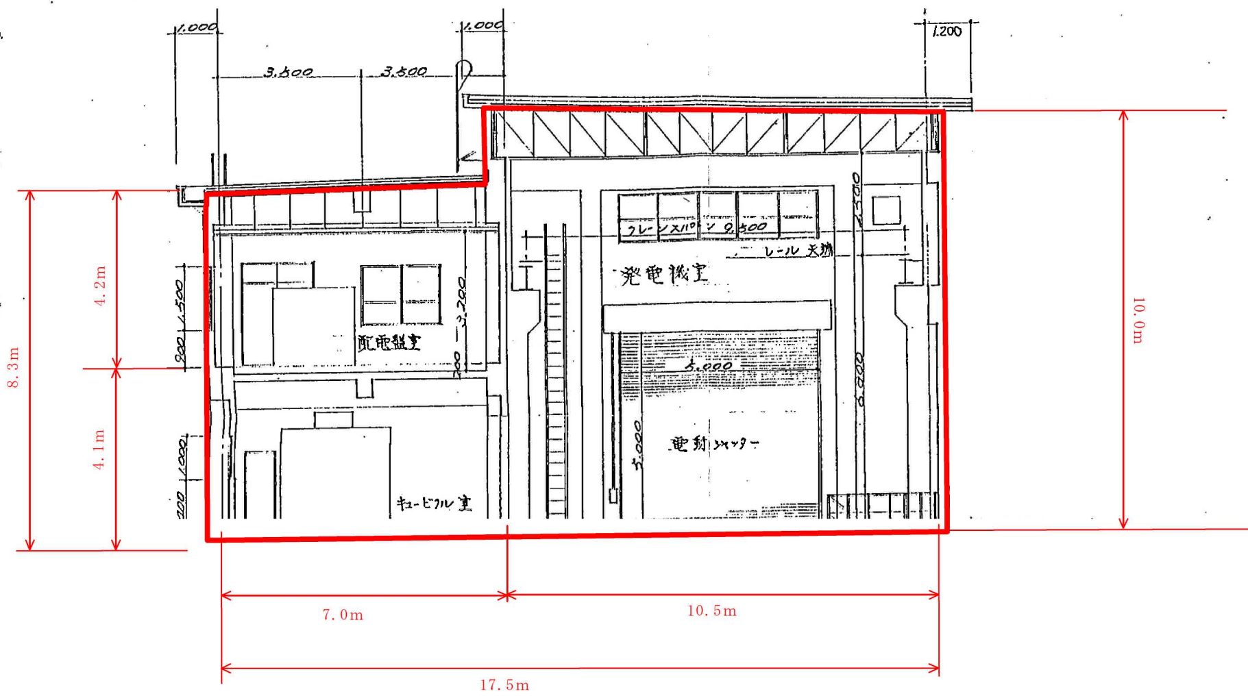
外壁薬剤散布範囲
