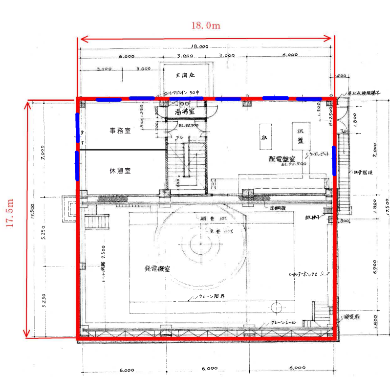
2階 平面図
