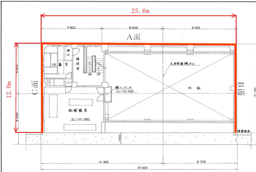
2階平面図
