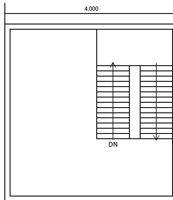
PH2階
