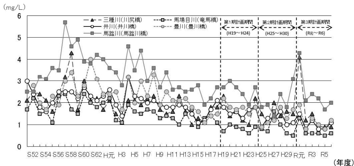
図 56 八郎湖流入河川の BOD（75%値）の経年変化
