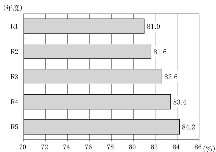
図 18 水洗化率の推移
