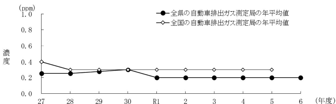
図37 一酸化炭素濃度の年平均値の経年変化
