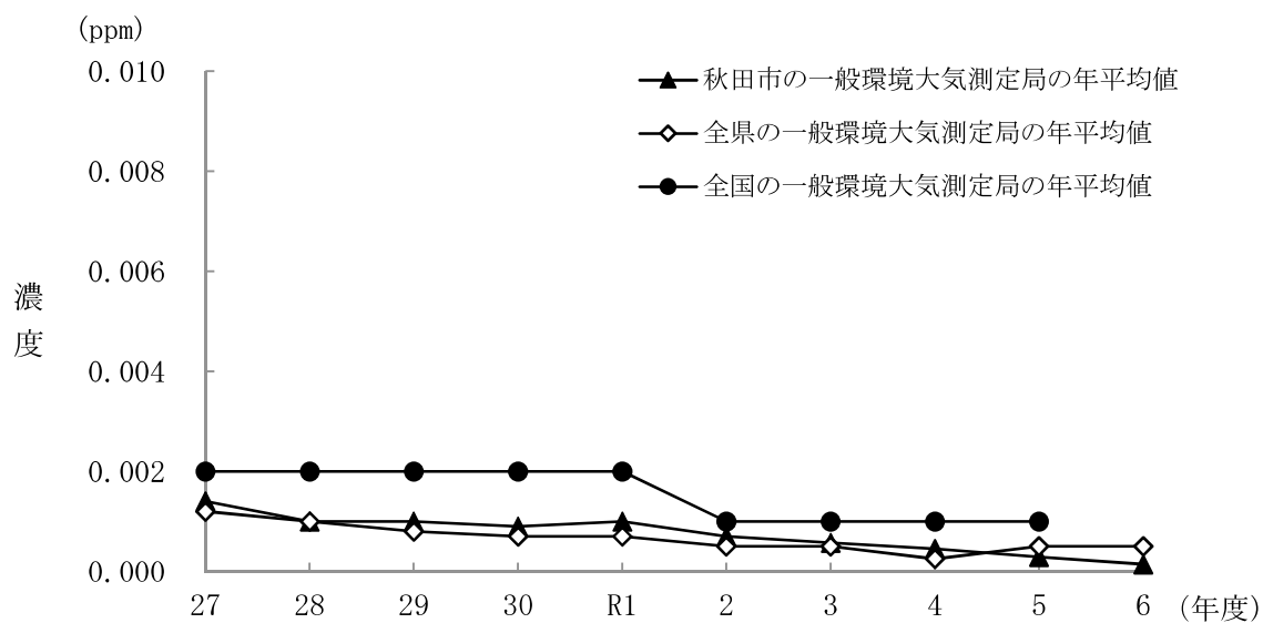
図30 二酸化硫黄濃度の年平均値の経年変化
