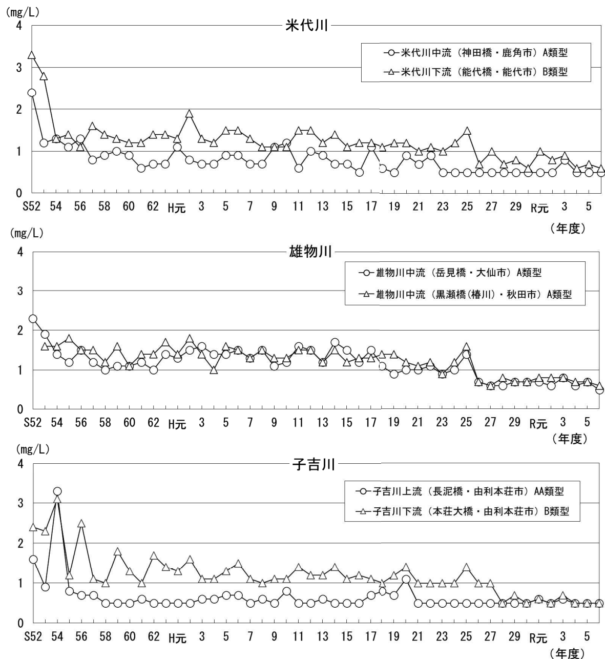
図 50 県内主要河川の BOD（75% 値）の経年変化
