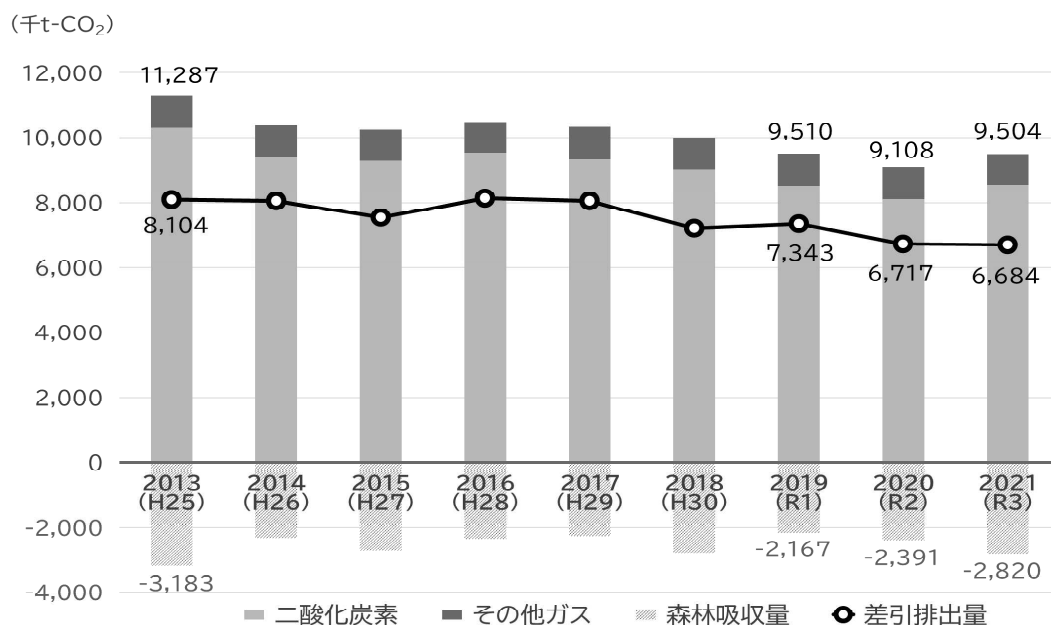
図 79 温室効果ガス排出量の推移
