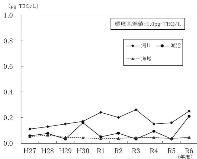
図 71 水質中の濃度推移（平均値）
