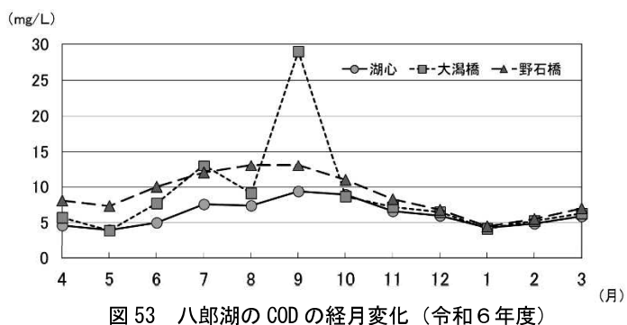
図 53 八郎湖の COD の経月変化（令和 6 年度）
