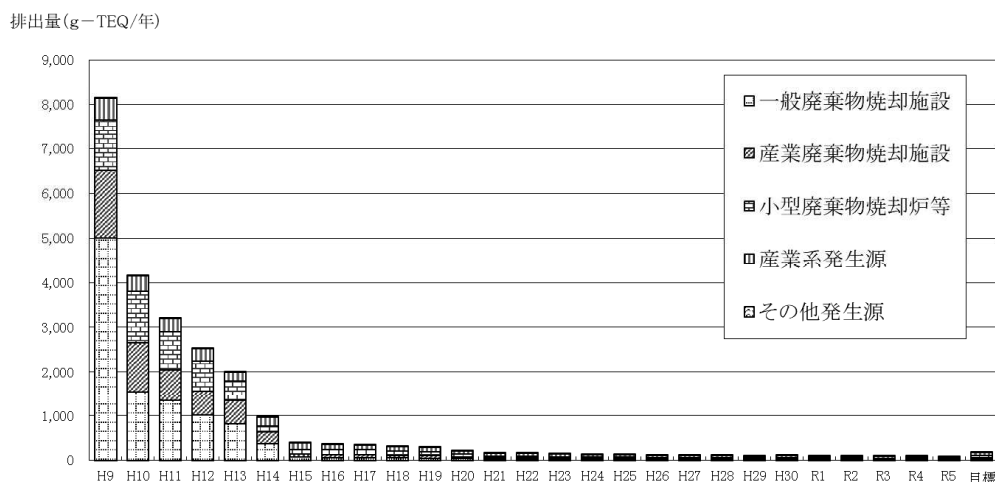
図 69 ダイオキシン類の排出総量の推移（全国）
