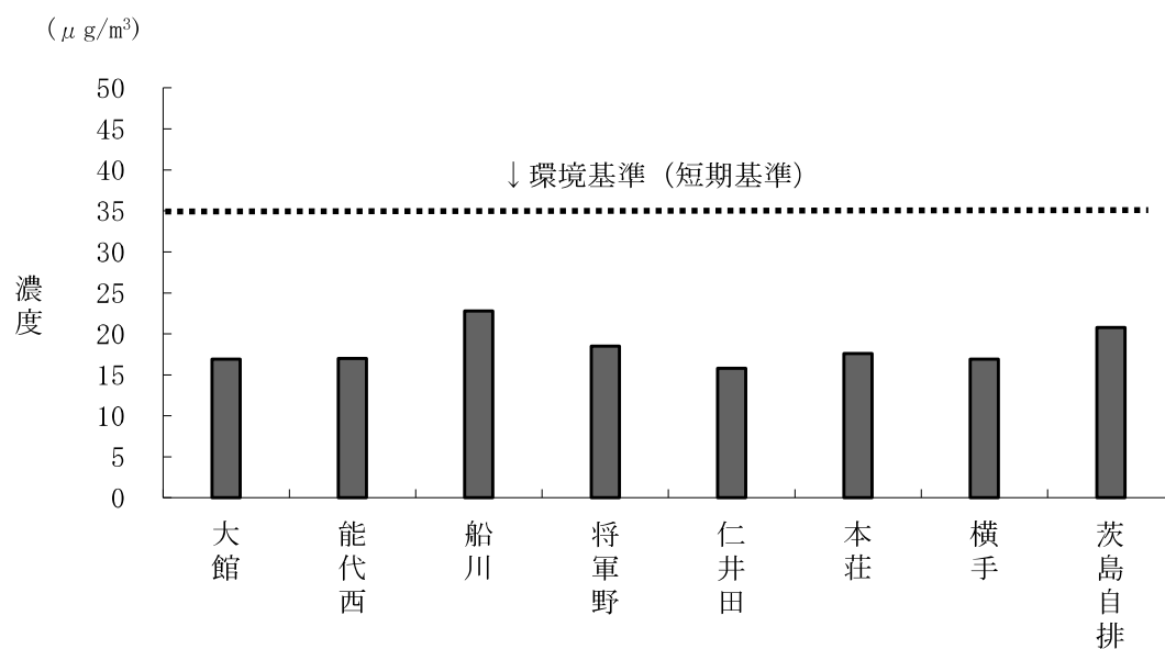
図44 微小粒子状物質の日平均値の年間98%値（令和6年度）
