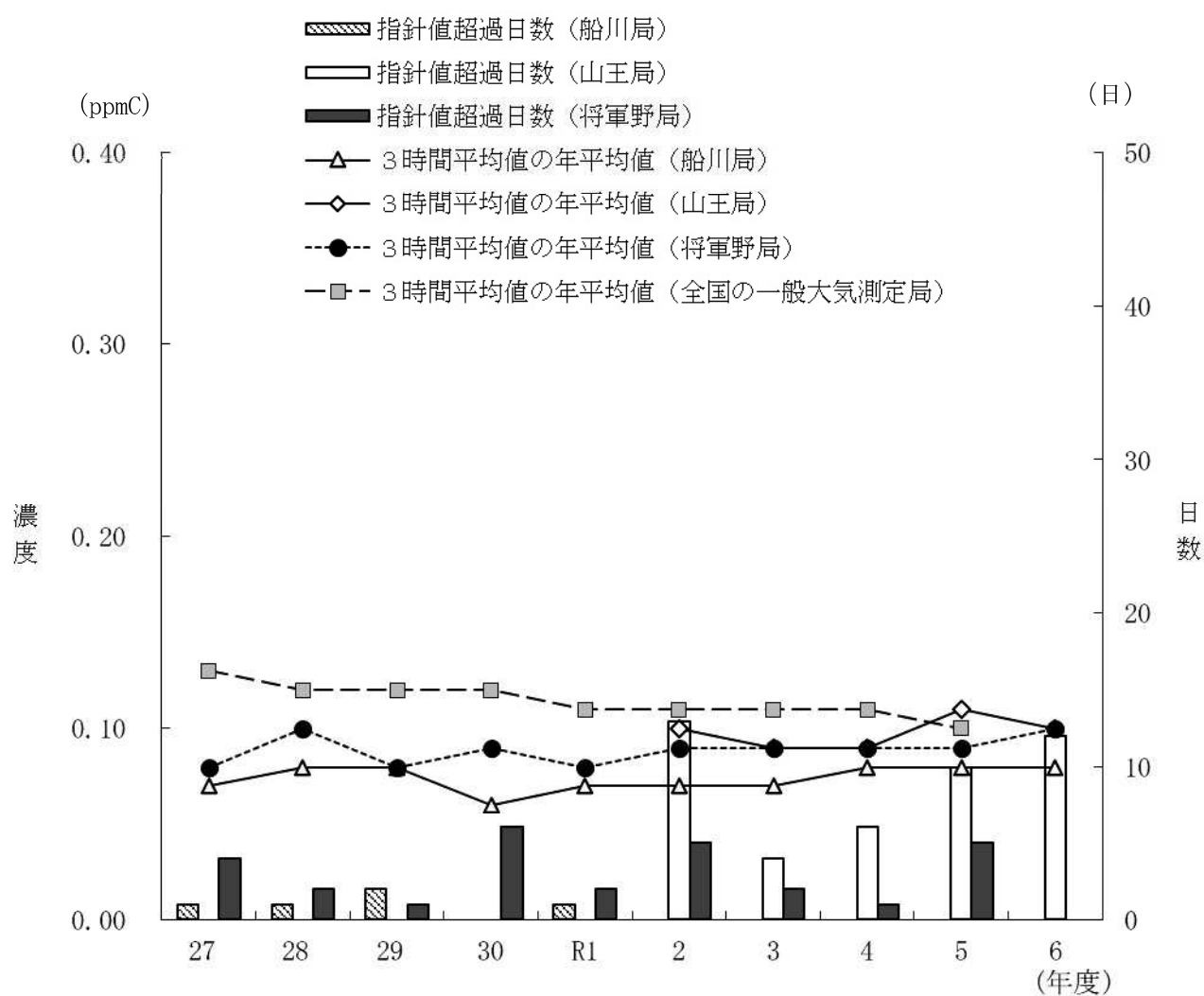
図47 非メタン炭化水素の3時間平均値及び指針値超過日数の経年変化
