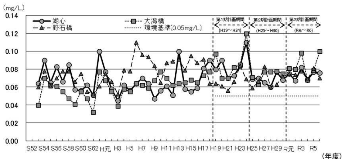
図 55 八郎湖の全りんの経年変化（表層、年平均値）
