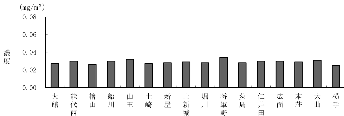
図41 浮遊粒子状物質の日平均値の年間2%除外値（令和6年度）
