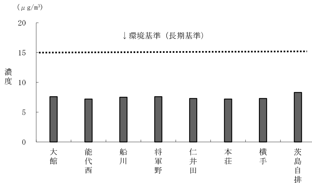
図43 微小粒子状物質の年平均値（令和6年度）
