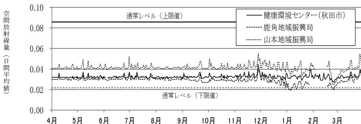
図 80 令和 6 年度の空間放射線量の推移（県中央から北部）
