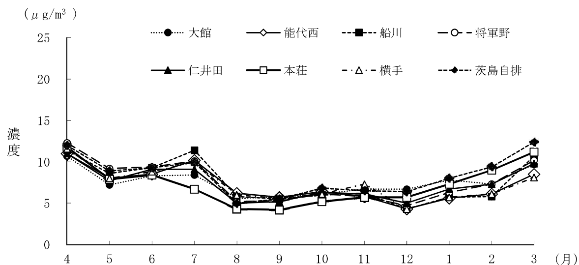
図45 微小粒子状物質の月平均値（令和6年度）
