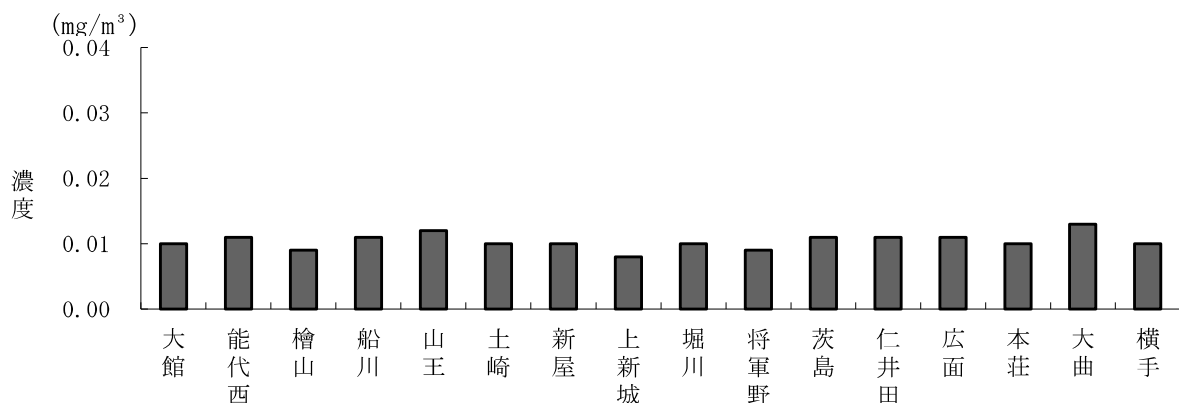
図40 浮遊粒子状物質の年平均値（令和6年度）
