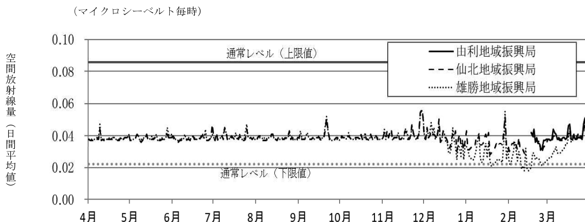
図 81 令和 6 年度の空間放射線量の推移 (県南部)
