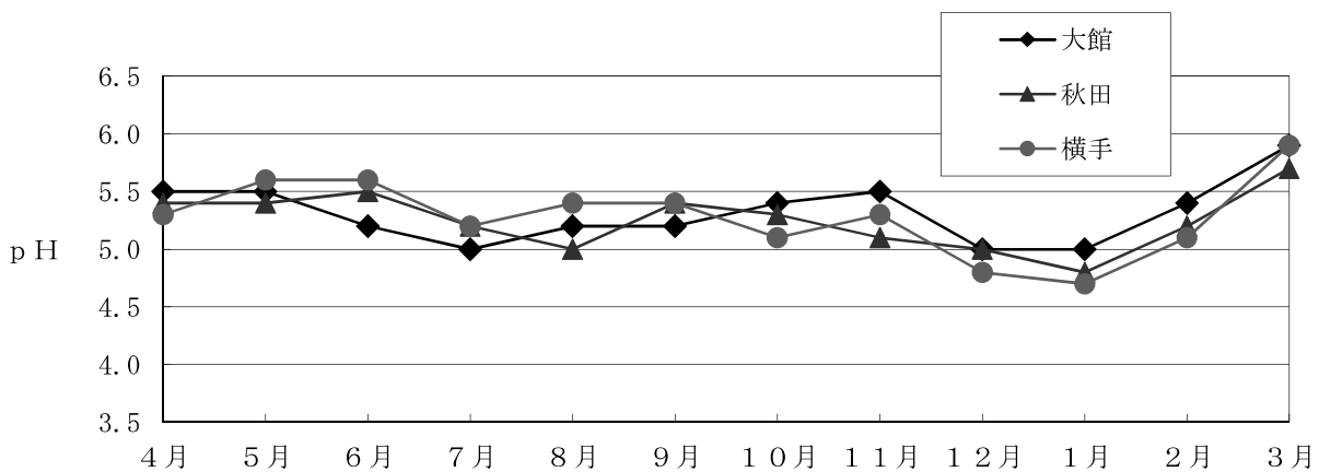
図 35 県内 3 地点における降雨・降雪の pH (月平均値) (令和 6 年度)
