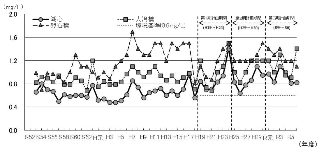
図 54 八郎湖の全窒素の経年変化（表層、年平均値）
