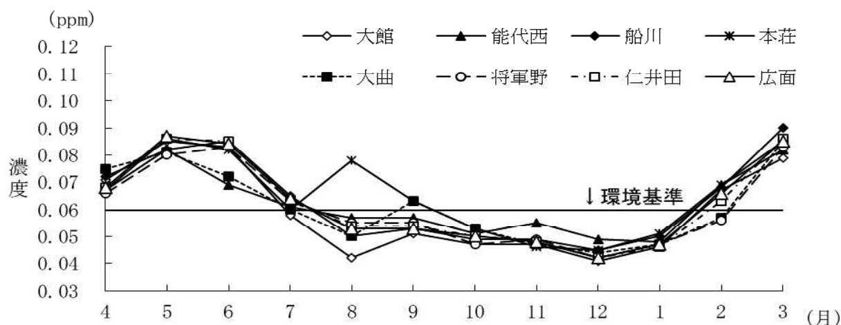
図38 光化学オキシダントの1時間値（昼間）の最高値の月別変化（令和6年度）
