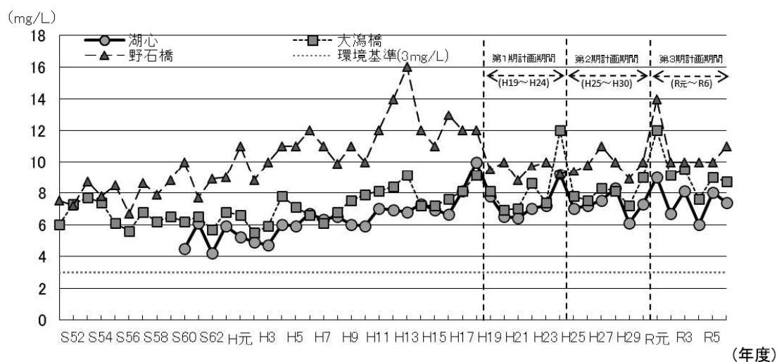
図 52 八郎湖の COD（75%値）の経年変化
