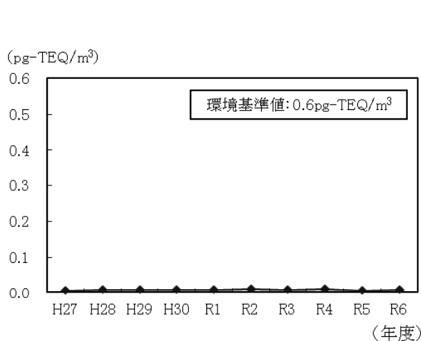
図 70 大気中の濃度推移（平均値）
