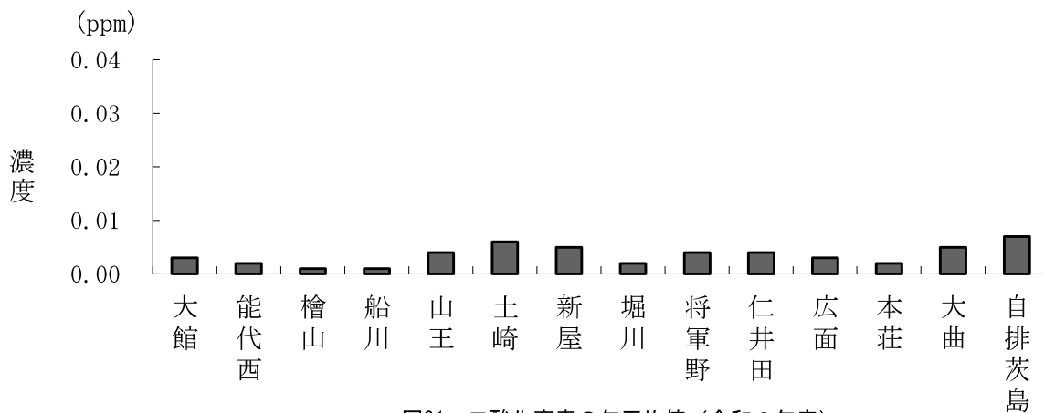
図31 二酸化窒素の年平均値(令和6年度)
