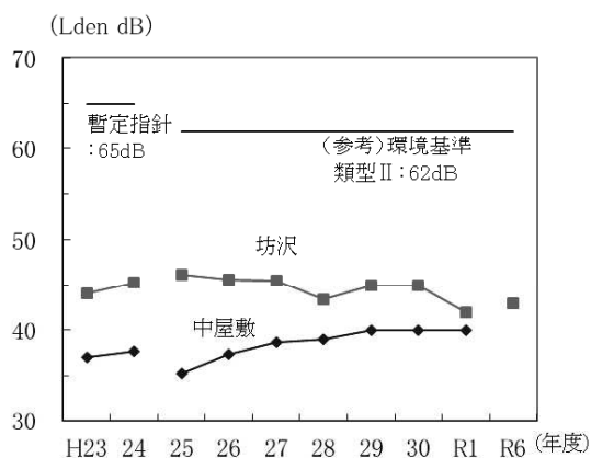
図 49 調査結果の経年変化（大館能代空港）
