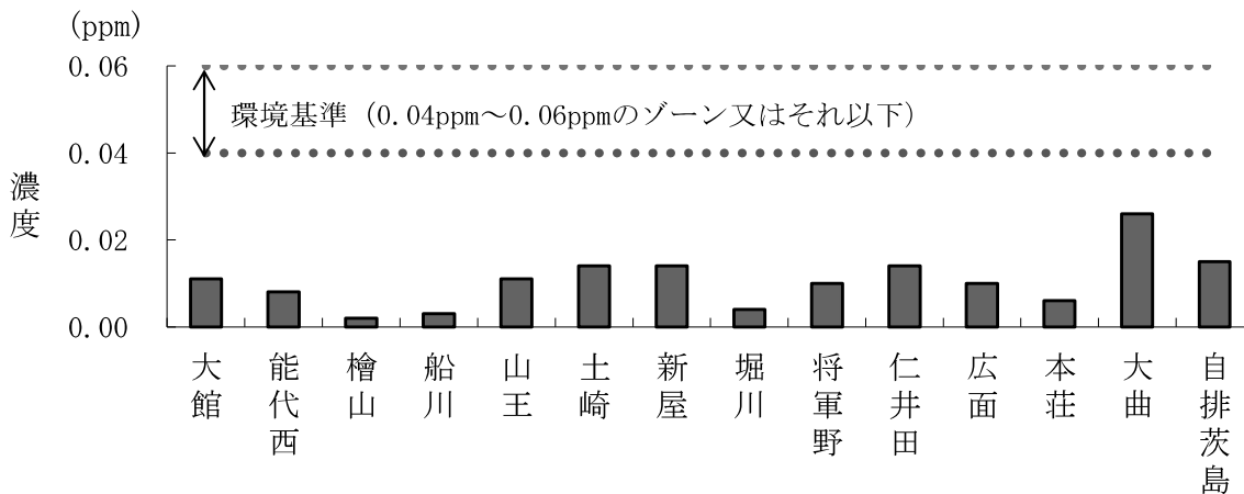
図32 二酸化窒素の日平均値の年間98%値(令和6年度)
