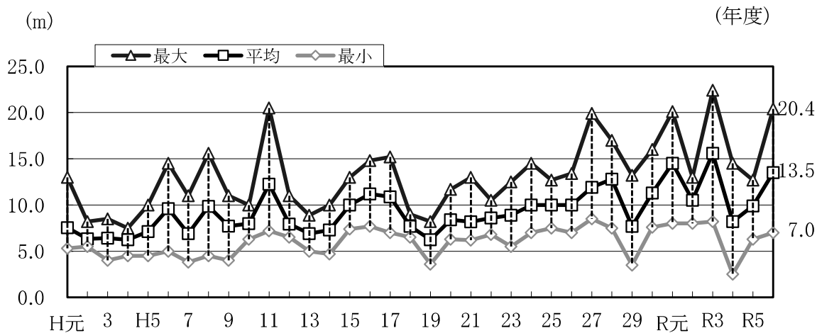
図 63 田沢湖（湖心）の透明度の経年変化
