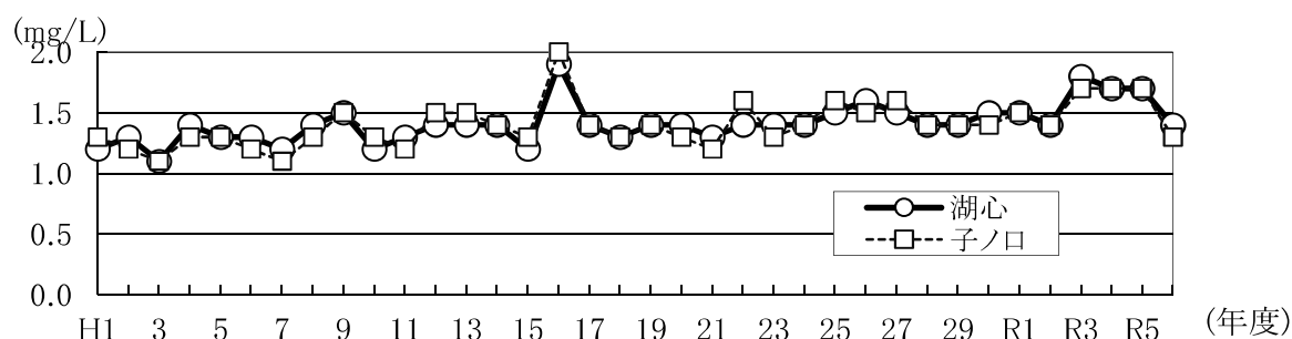
図 58 十和田湖の COD（75% 値）の経年変化
