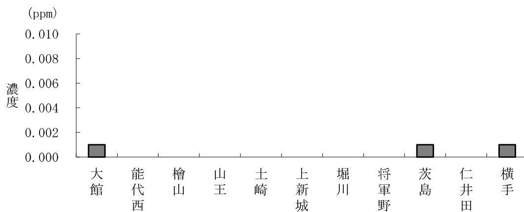
図28 二酸化硫黄の年平均値 (令和 6 年度)
