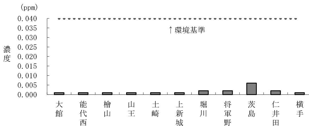
図29 二酸化硫黄の日平均値の年間 2 %除外値 (令和 6 年度)
