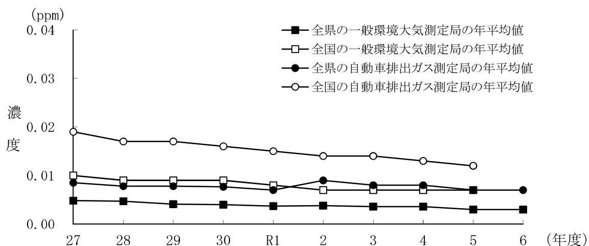
図33 二酸化窒素濃度の年平均値の経年変化
