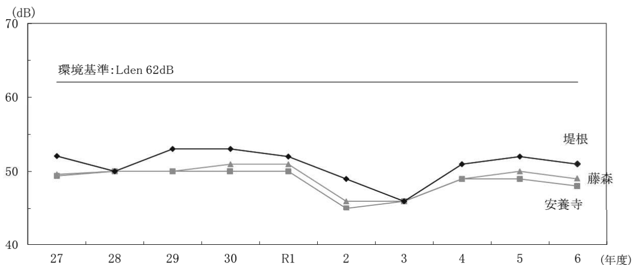
図 48 調査結果の経年変化（秋田空港）
