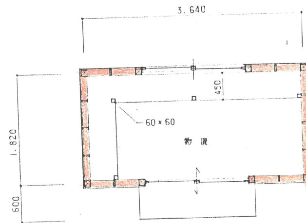
平面図 S = 1 : 50
