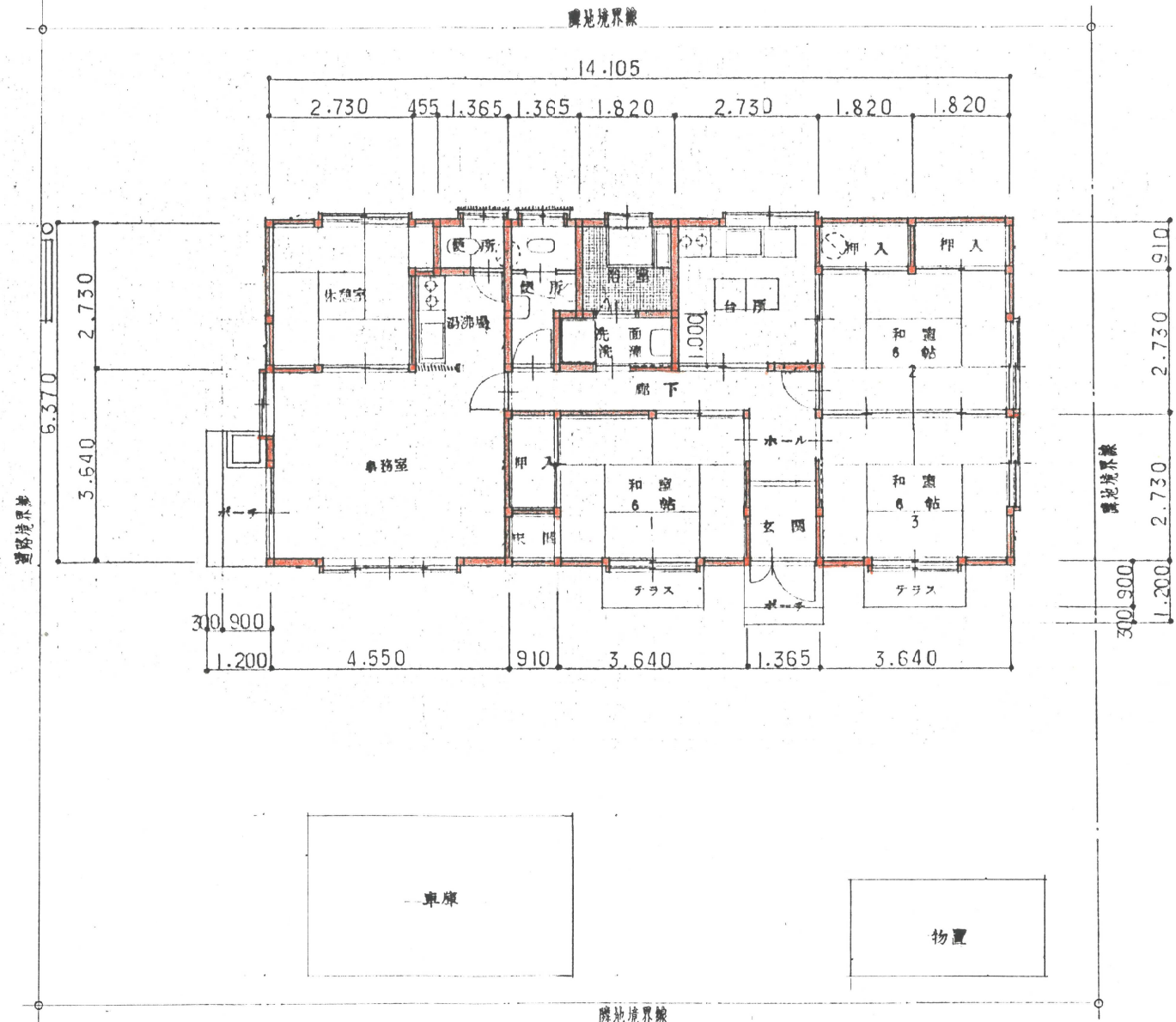
配置平面図 S-1:100
