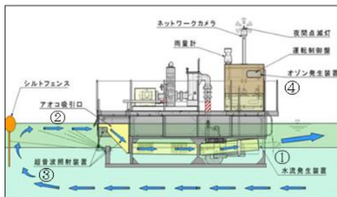
図 36 アオコ抑制装置側面図
