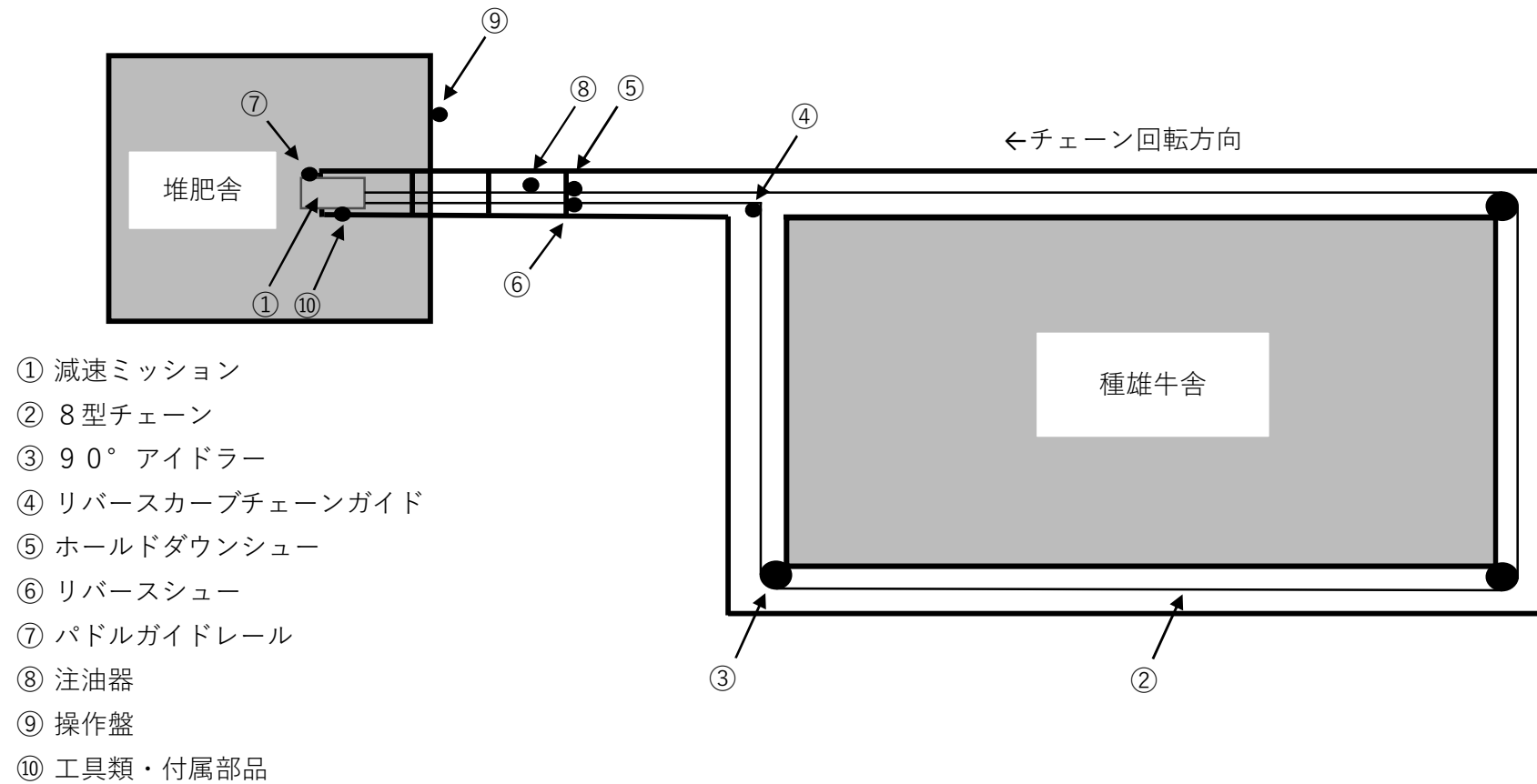
秋田県畜産試験場種雄牛舎バンクリーナー配置図
