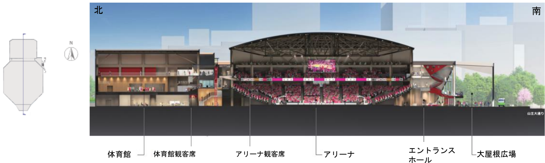
内観透視図
