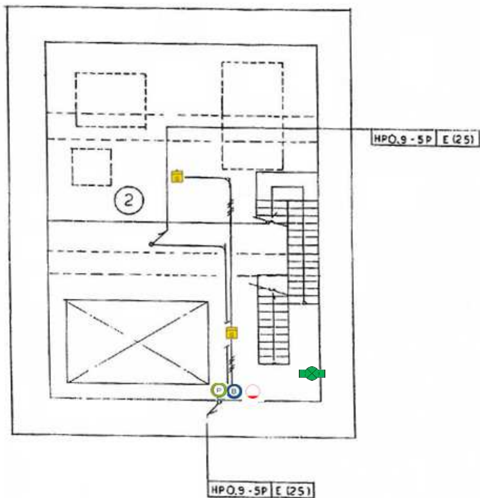
地下1階平面図
