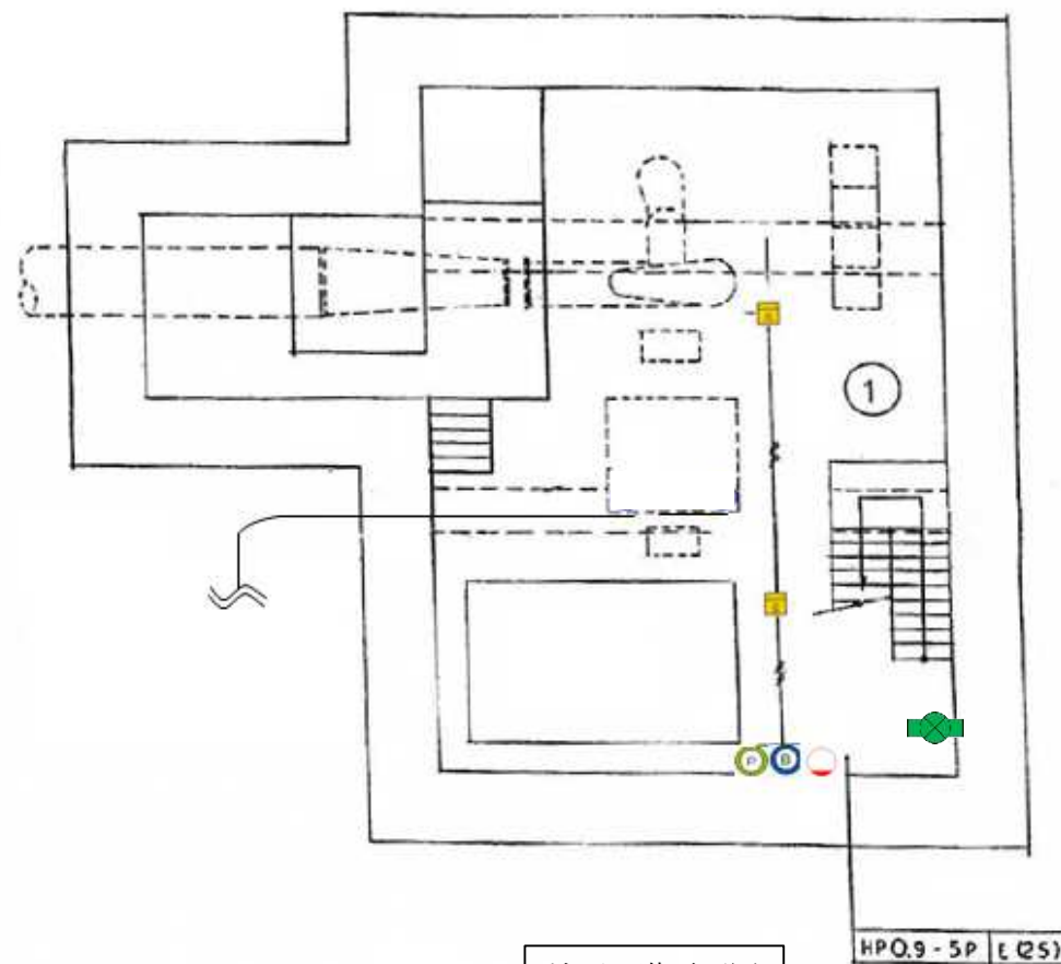
地下2階平面図
