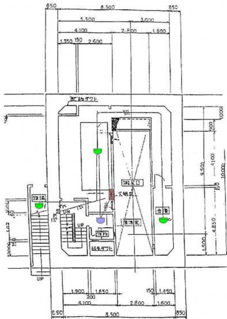
配電盤室
