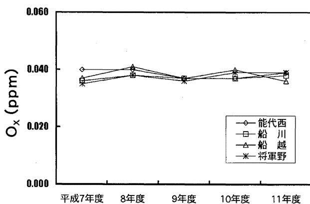
図8 光化学オキシダント昼間の1時間値の年平均値の推移
