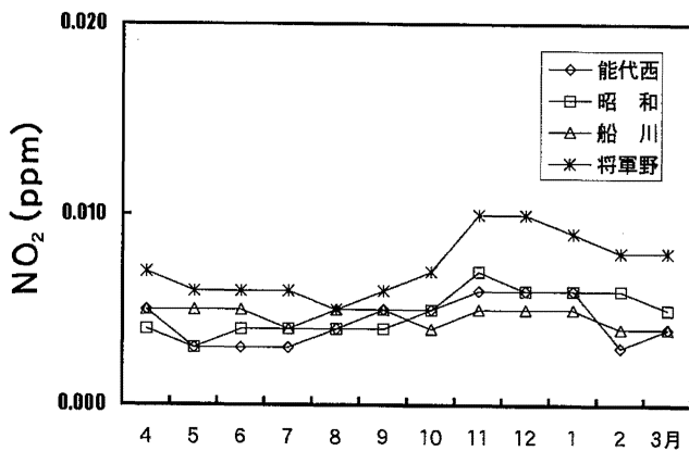
図7 主要測定局での二酸化窒素月平均値の変化
