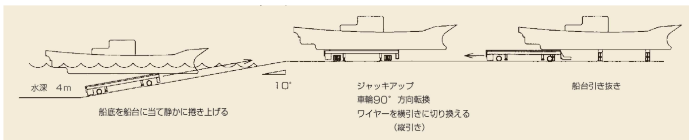
〔漁船上架施設の模式図〕
