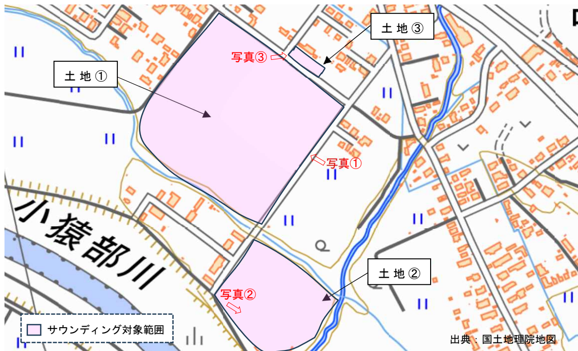
○配置図
