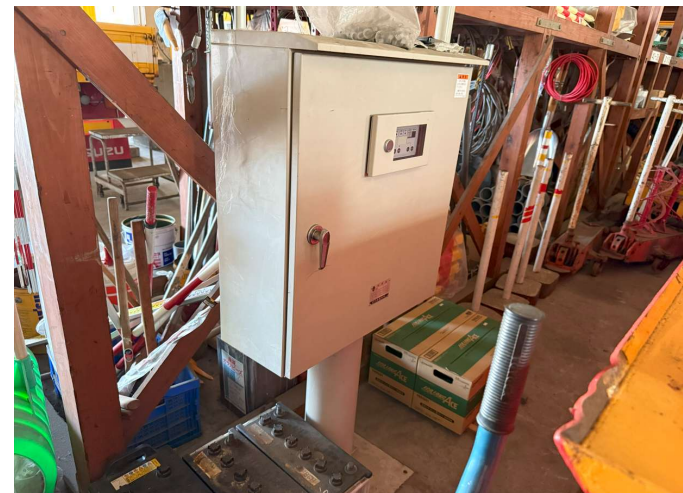
NO.23 積雪センサー制御盤
