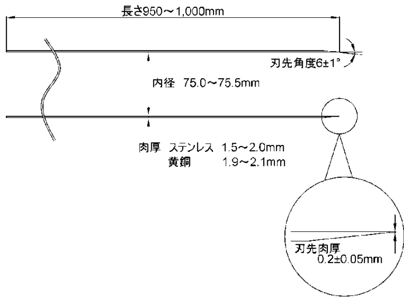
図7-1 サンプリングチューブ
