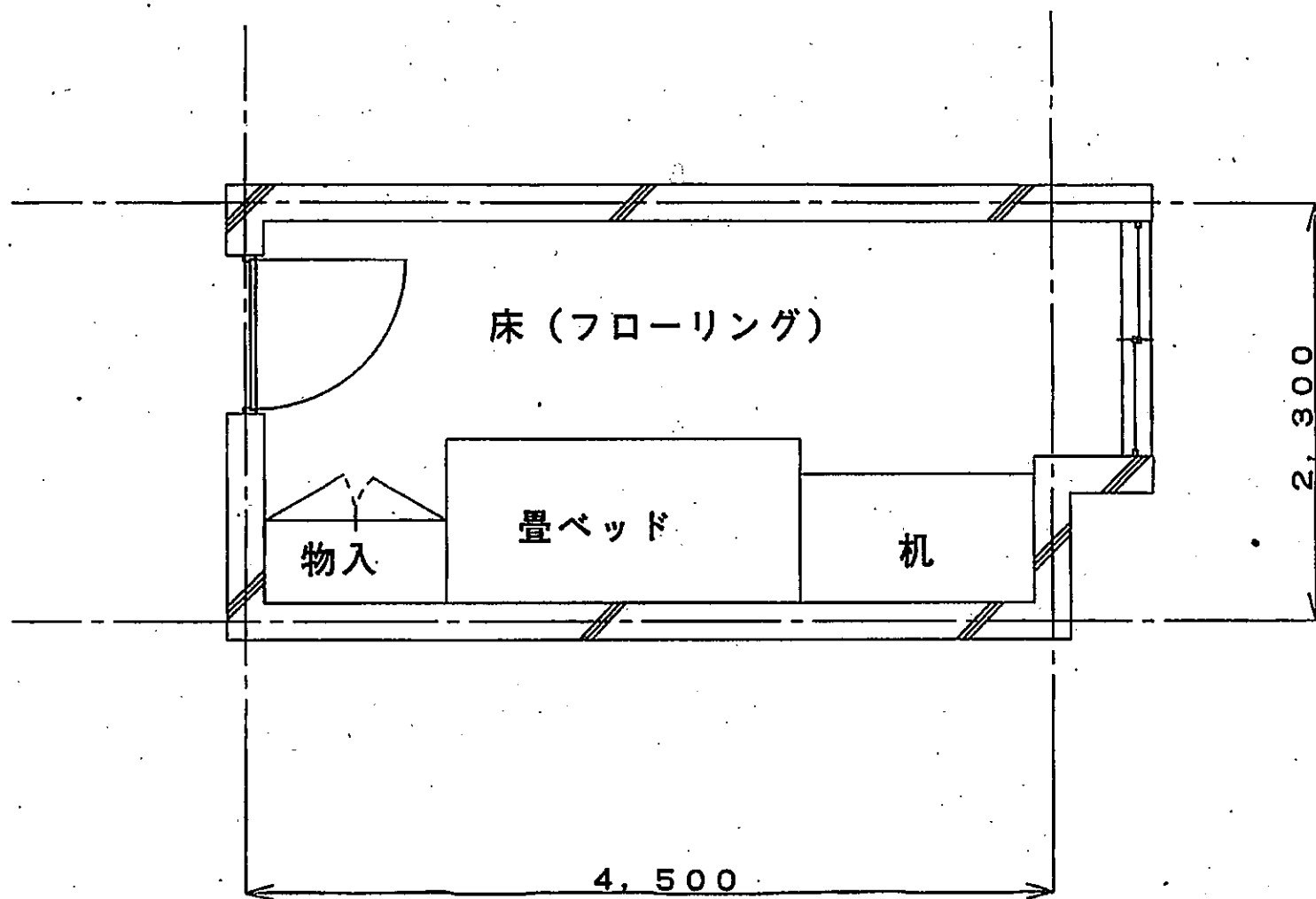
学生寮平面図
