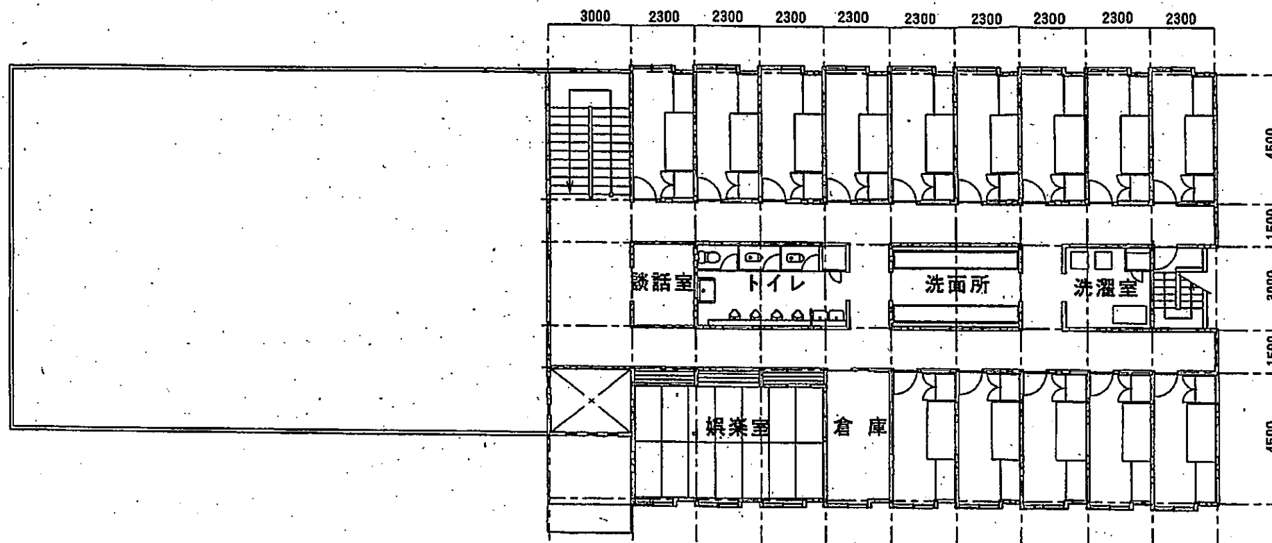
清和寮 2階平面図
