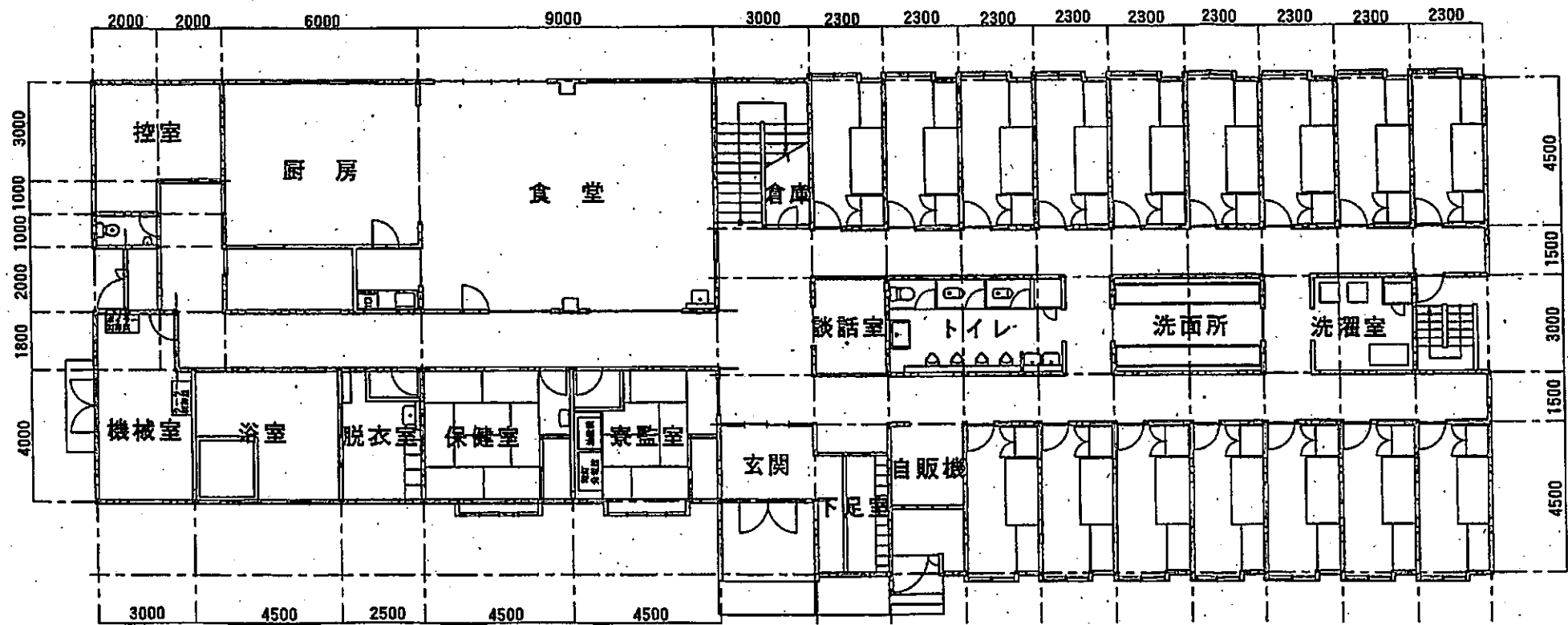
清和寮 1階平面図
