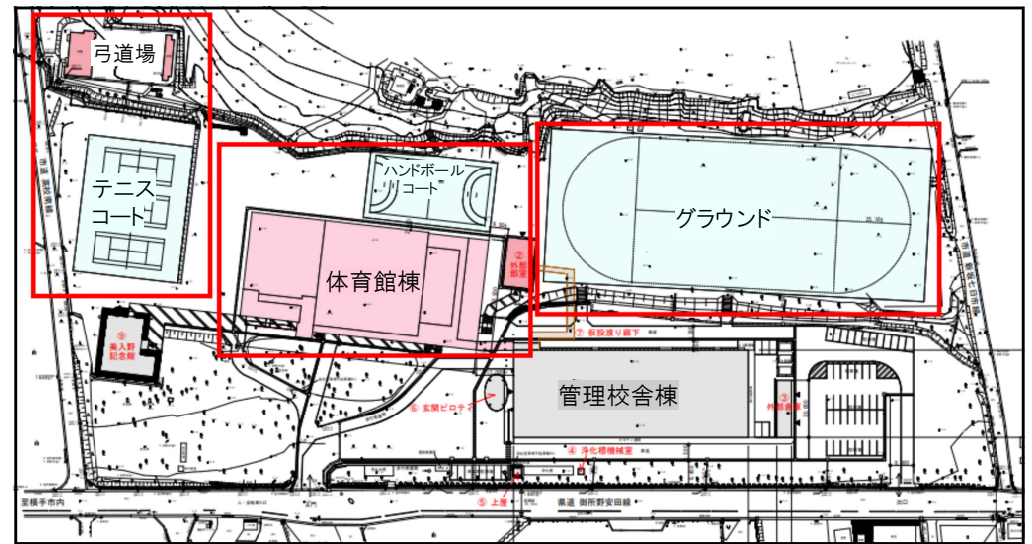
○配置図
