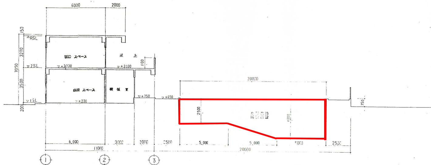
断面图 SCALE: 100
