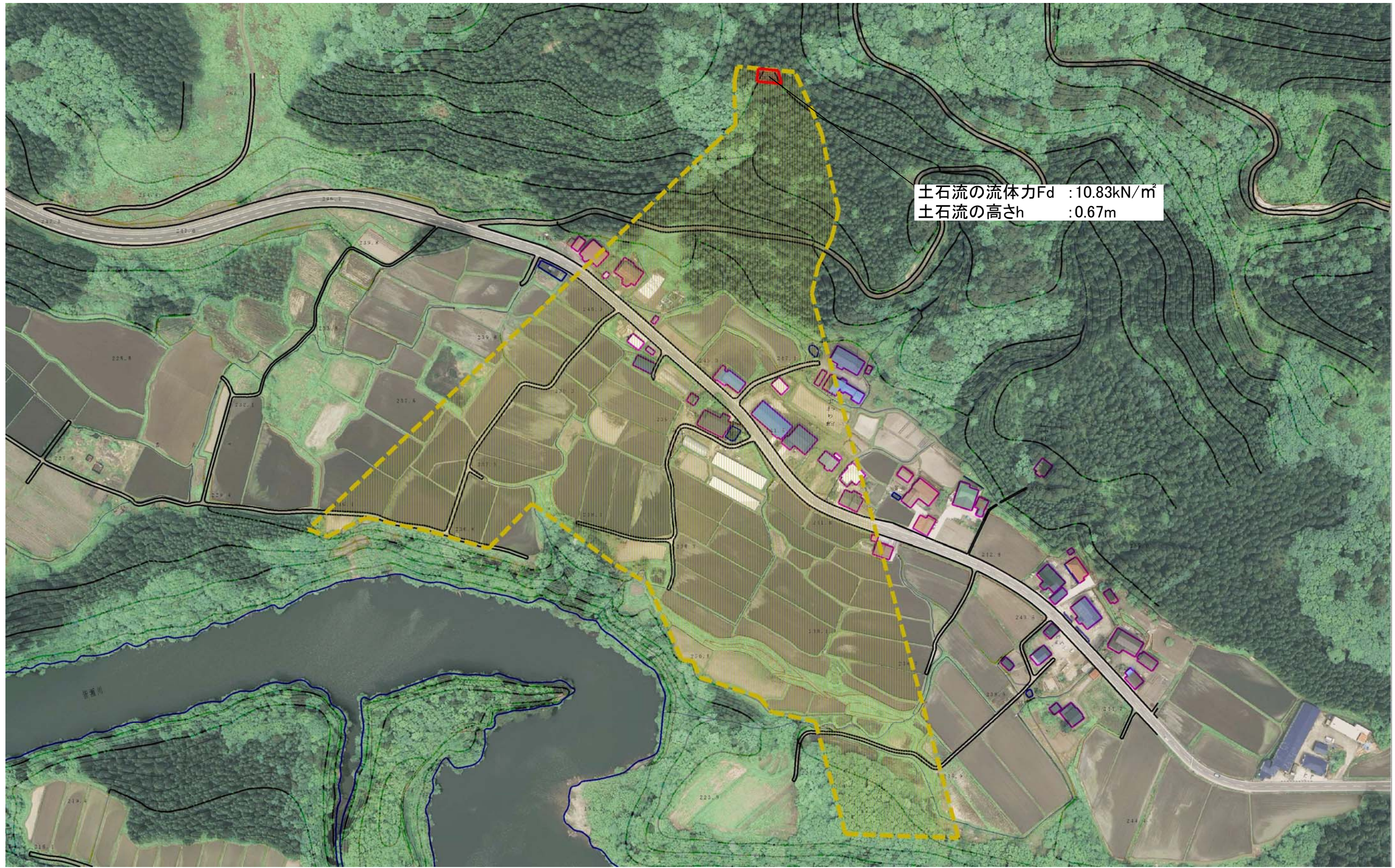
様式-2(土) 土砂災害警戒区域・土砂災害特別警戒区域 区域図(その2)
