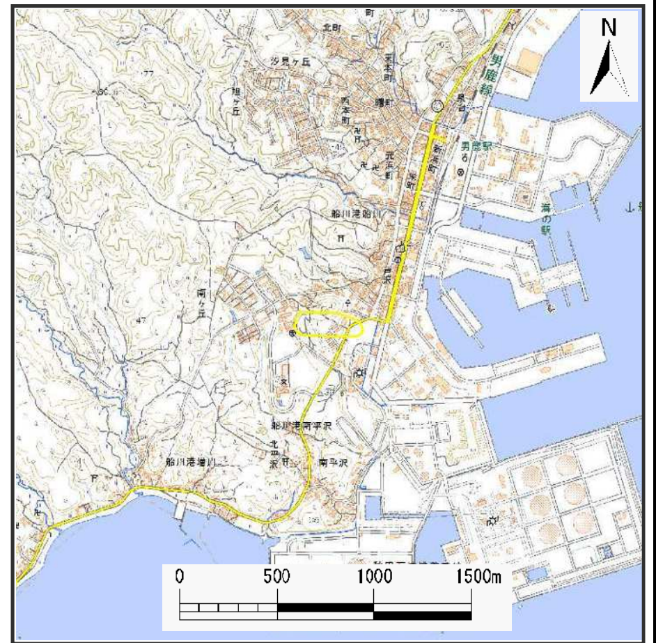
位置図 (S=1:25,000)
