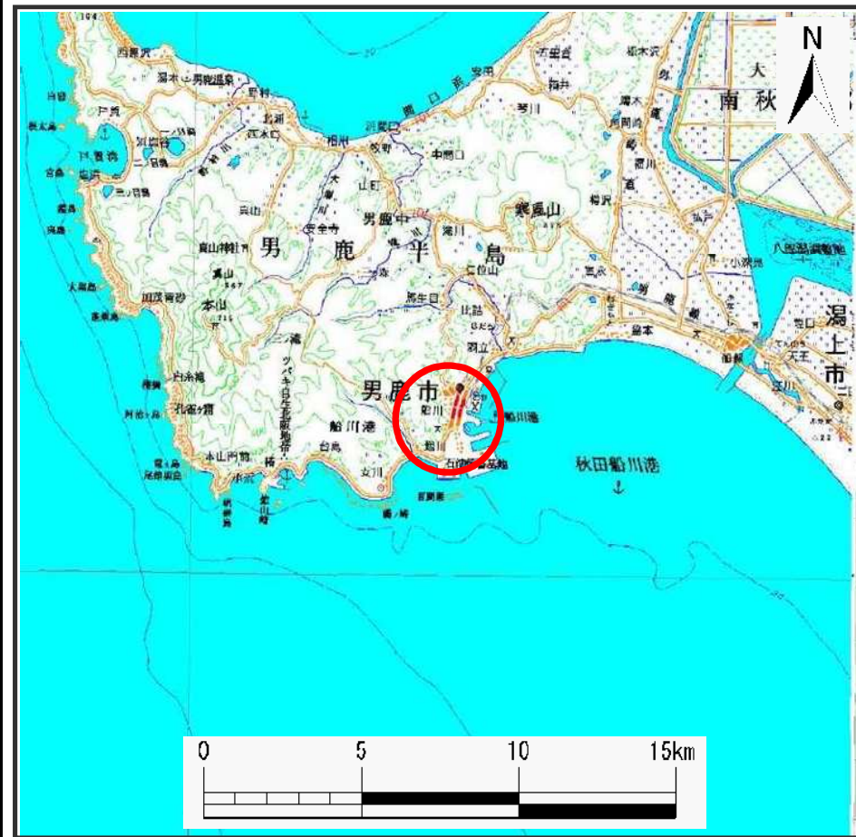
位置図 (S=1:200,000)
