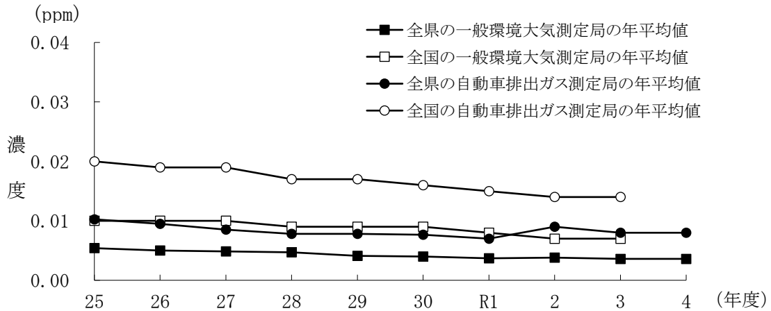
図31 二酸化窒素濃度の年平均値の経年変化
