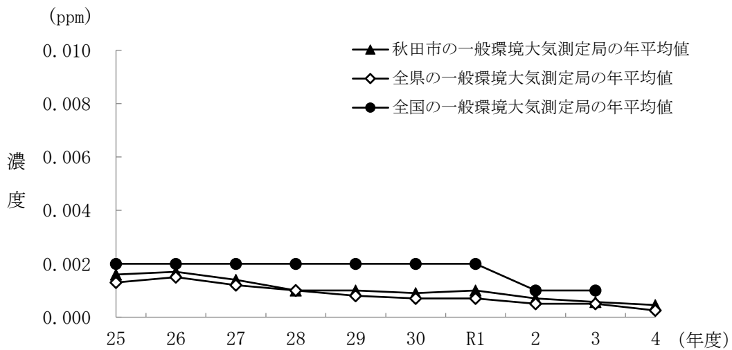
図31 二酸化硫黄濃度の年平均値の経年変化
