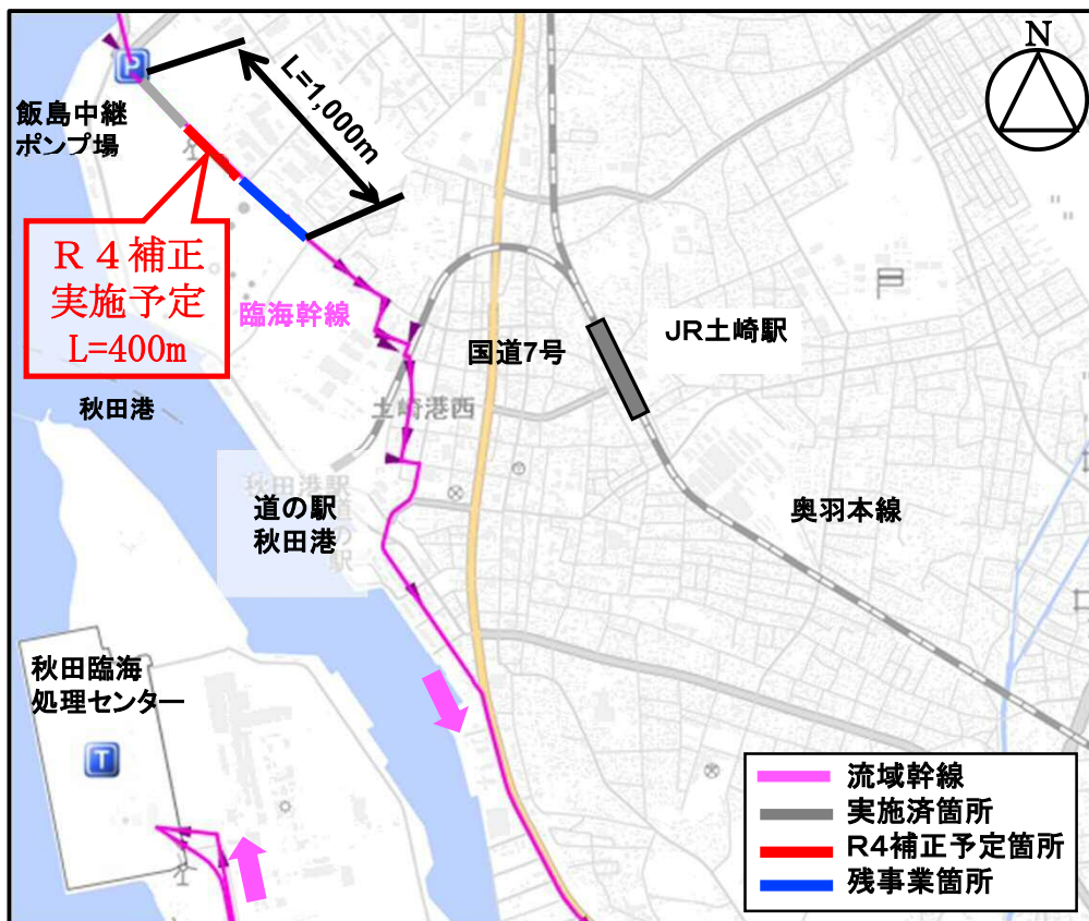
臨海処理区 臨海幹線 (秋田市)
