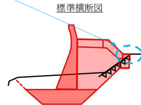
護岸工更新
