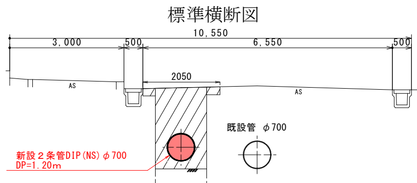
臨海処理区 臨海幹線 (秋田市)
