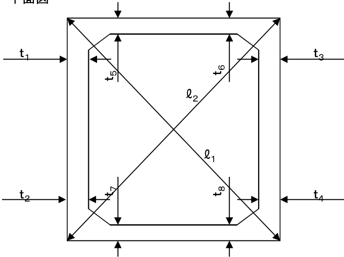
平面図
