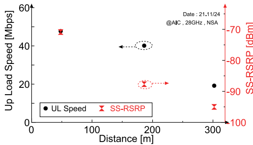
ミリ波5G距離と通信速度
