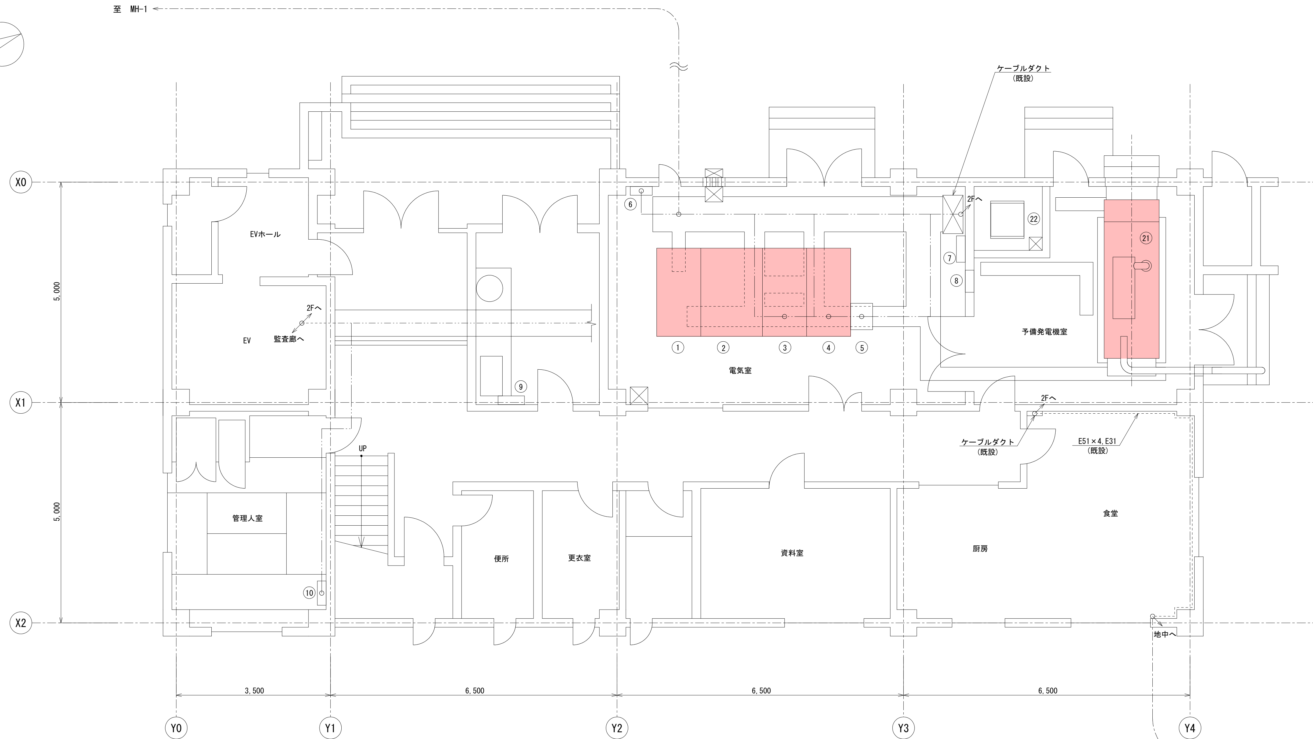
電気室上部平面図 S=1:50
