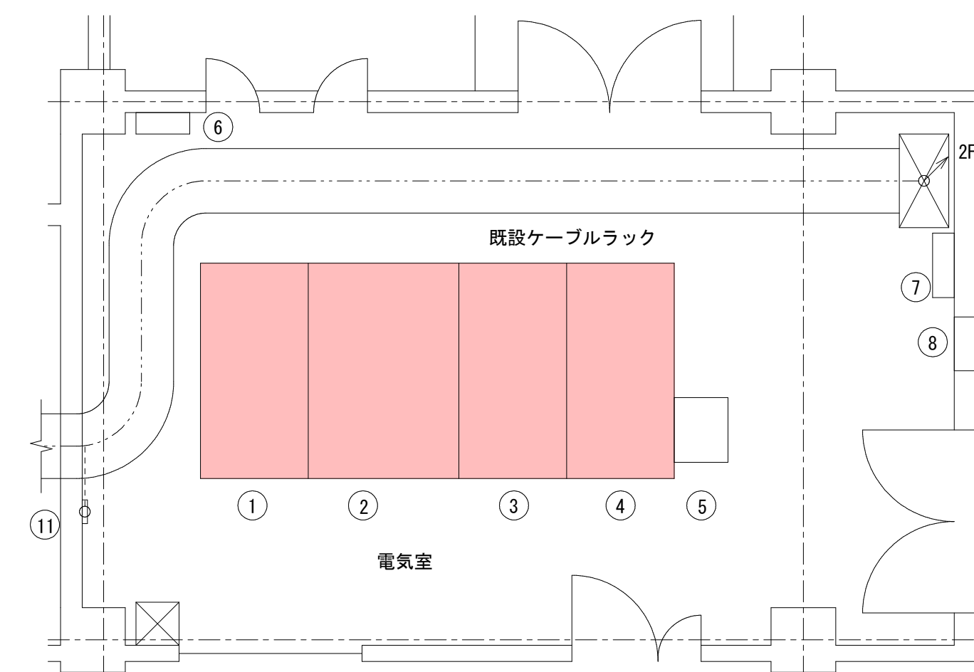
電気室上部平面図 S=1:50
