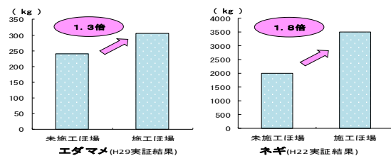
＜図＞地下かんがいシステムによる収量の向上
