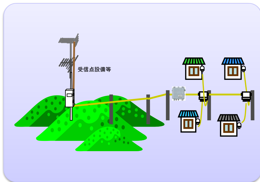
有線共聴
