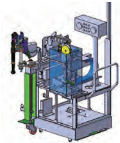
サスペンションリンク締付機 (3D-CADモデル)
