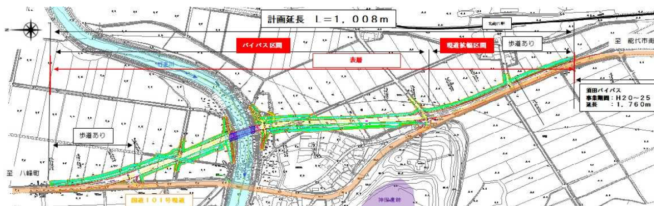
竹生バイパス 平面図
