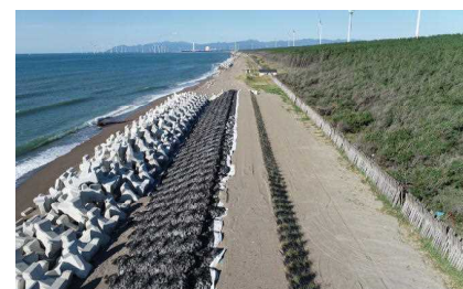
飛砂防備保安林を保全する防潮工
