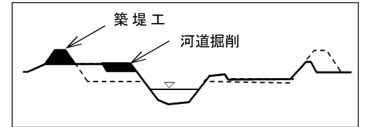
河道掘削、築堤工 標準横断面図
