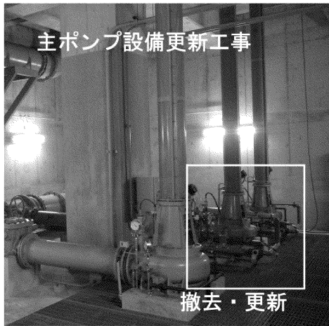
大曲中継ポンプ場（大仙市）
