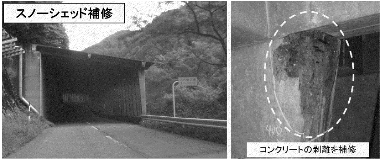
国道105号 ばんないもり 万内森2号スノーシェッド（北秋田市）
