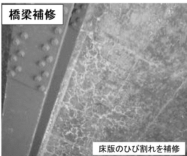
国道105号 馬橋（仙北市）
