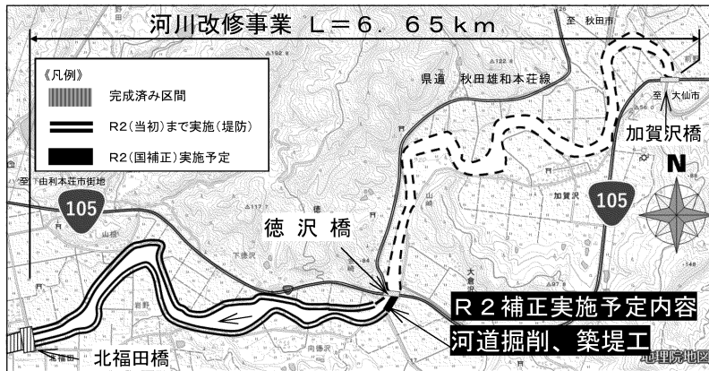
芋川（由利本荘市）
