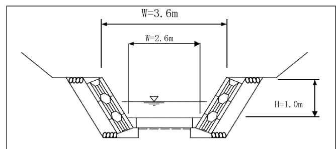
溪流保全工標準横断面図
