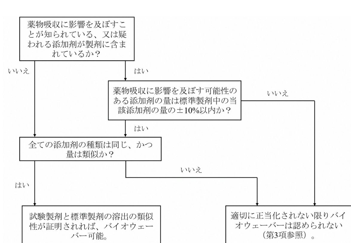
図 2. BCS クラス III の原薬
