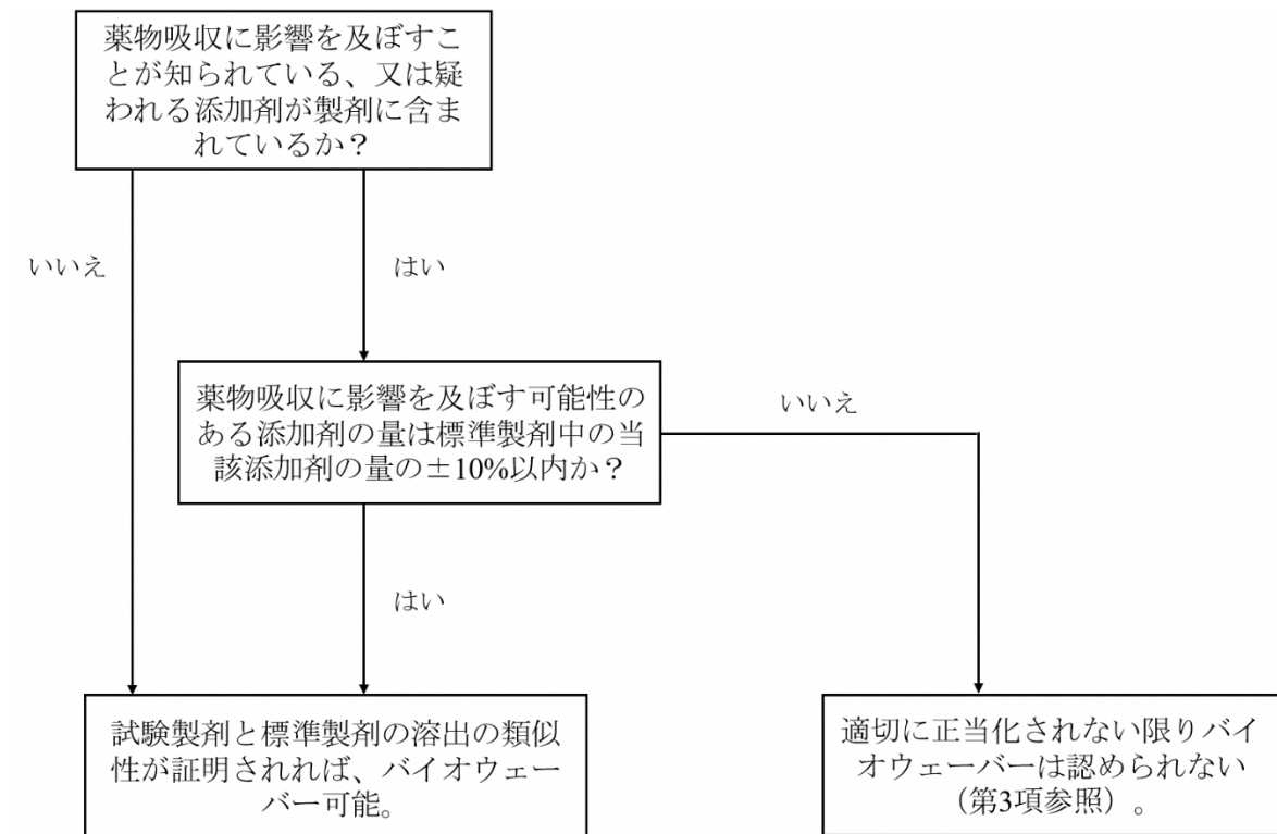
図 1. BCS クラス I の原薬
