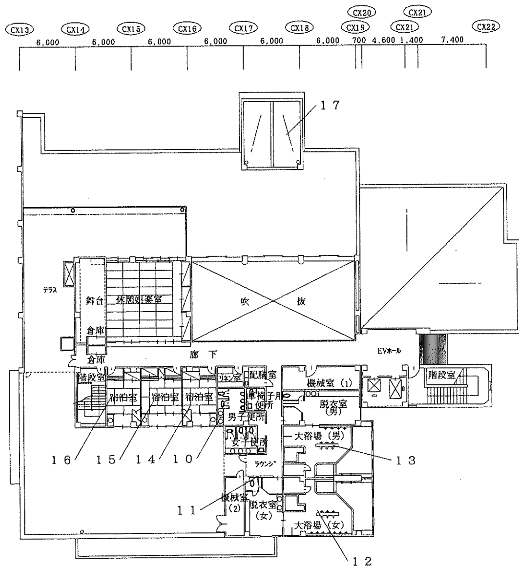
コミュニティセンター 2階平面図 S=1:400
