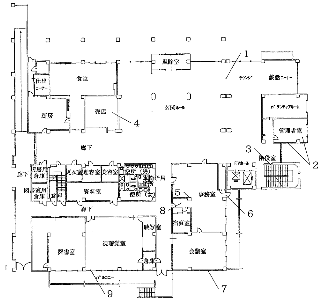
コミュニティセンター 1階平面図 S=1:400
