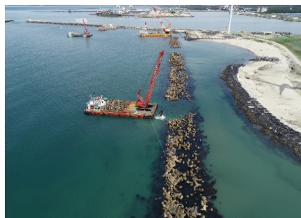
防波堤改良工事
