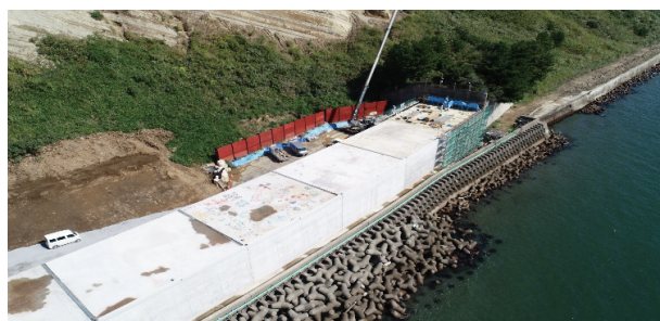
カルバート工
