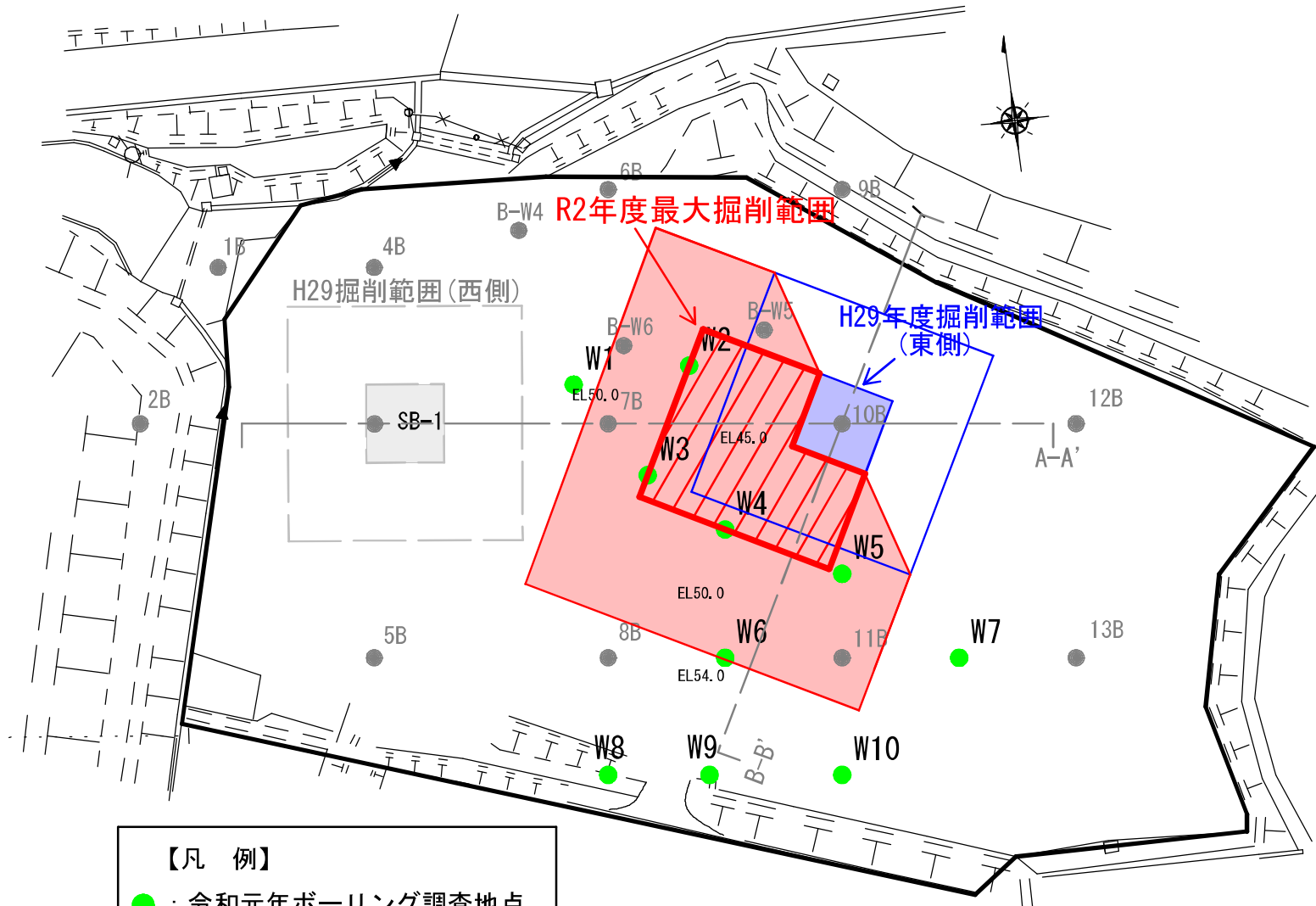
平面図
