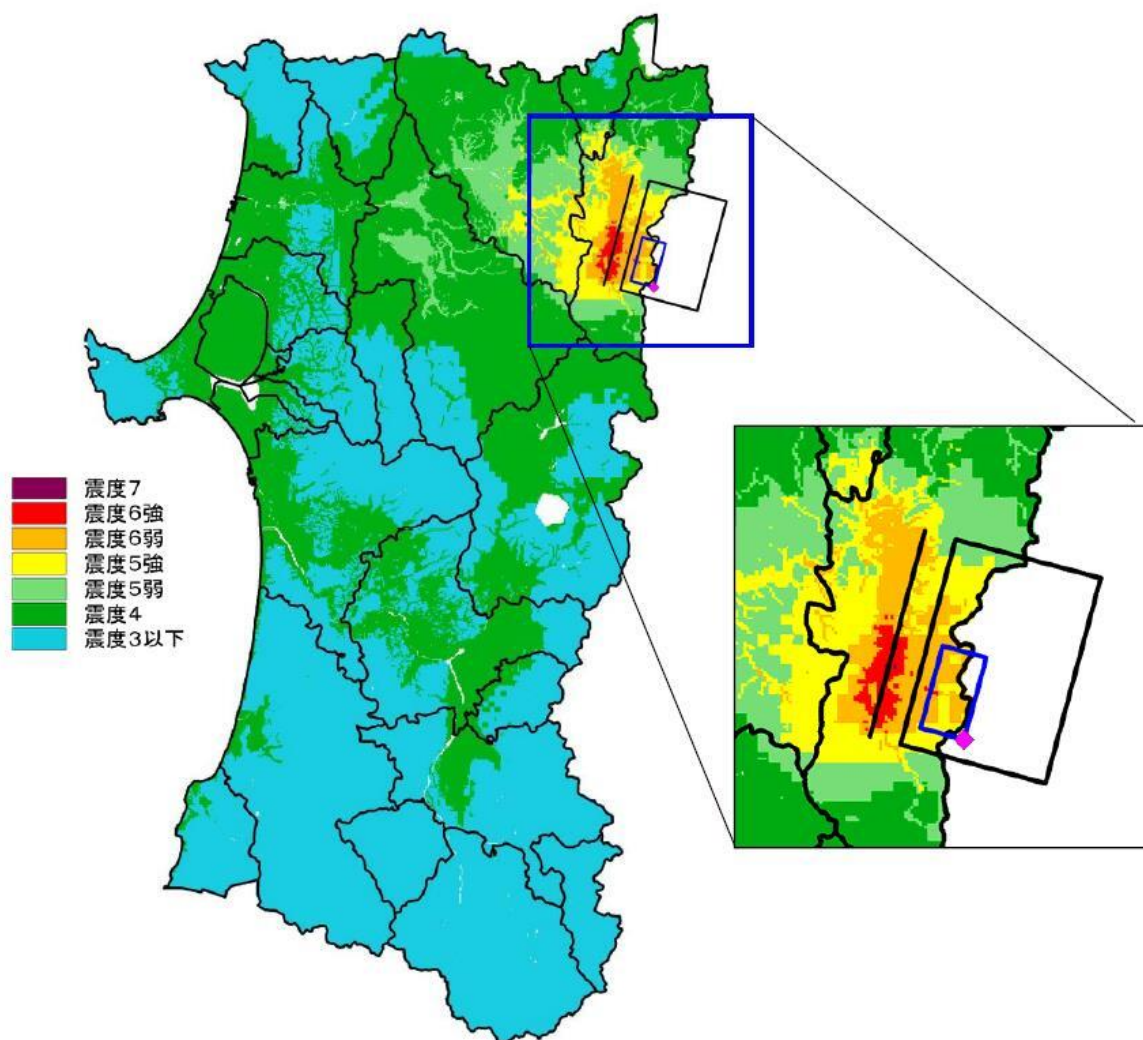
図-4.5.2 震度分布図（詳細法）
