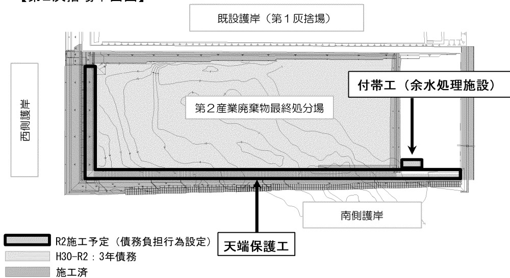
【第2灰捨場平面図】
