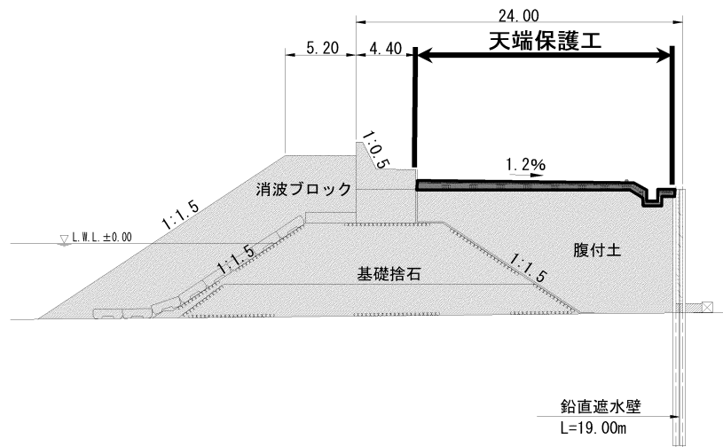
【南側護岸断面】
