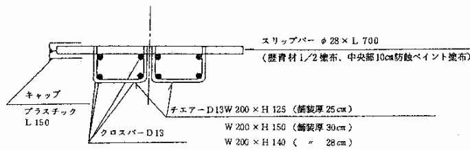
図-4 膨張目地
