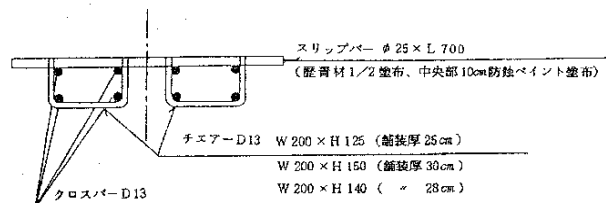
横収縮目地
