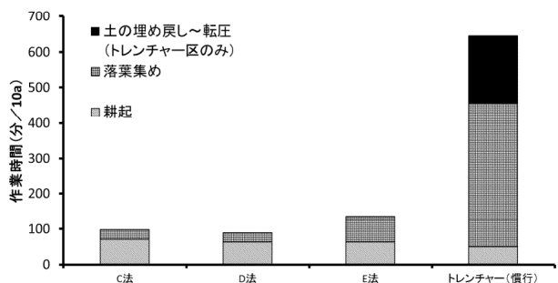
図1 各落葉処理方法による10a当の作業時間（平成28～29年）
