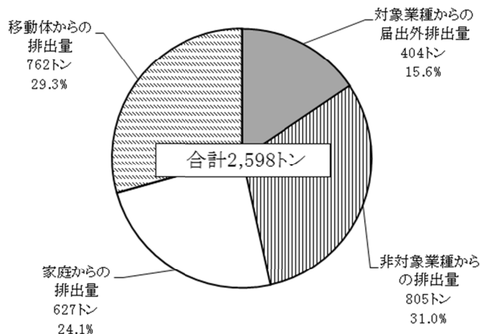
図9 届出外排出量内訳
