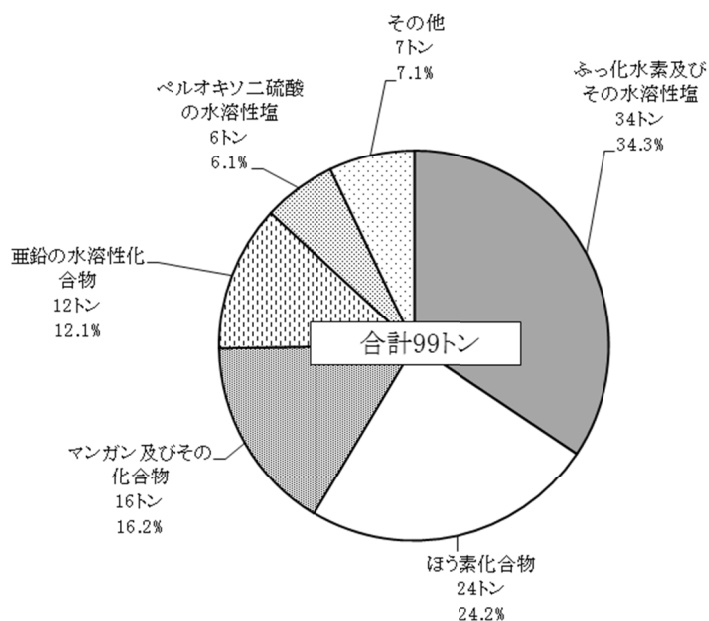
図4 公共用水域への排出量上位5物質
