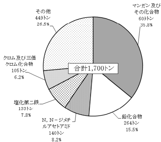
図8 届出移動量上位5物質
