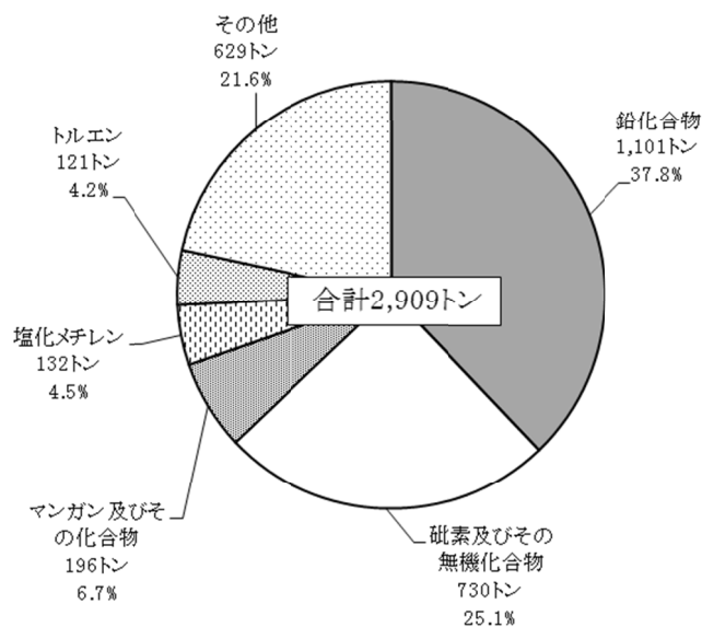
図6 届出排出量合計上位5物質
