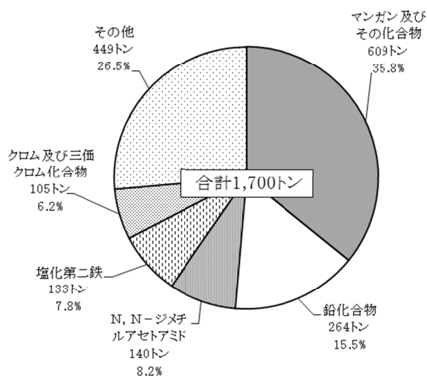
図7 事業所外への移動量上位5物質
