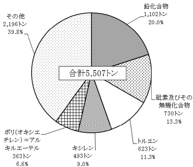
図10 届出排出量及び届出外排出量合計上位5物質
