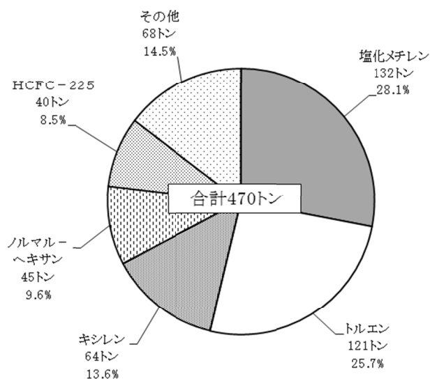
図3 大気への排出量上位5物質
