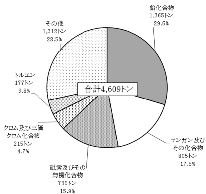
図2 排出量・移動量合計上位5物質
