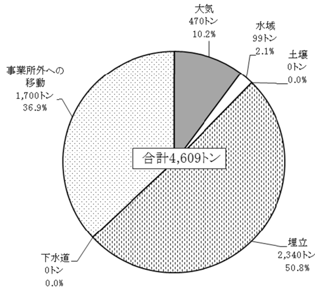
図1 排出量・移動量合計
