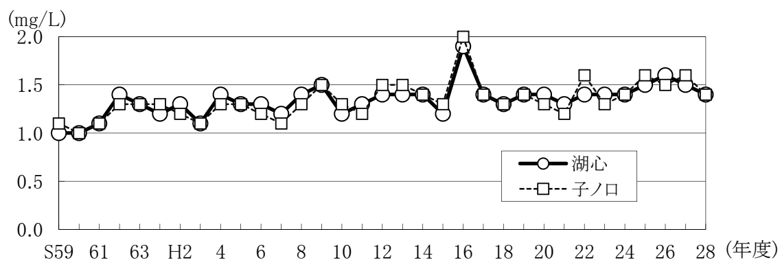
図43 十和田湖のCOD（75%値）の経年変化
