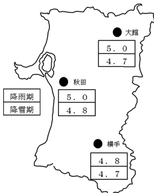
図81 県内3地点における降雨・降雪のpHの年平均値（平成28年度）
