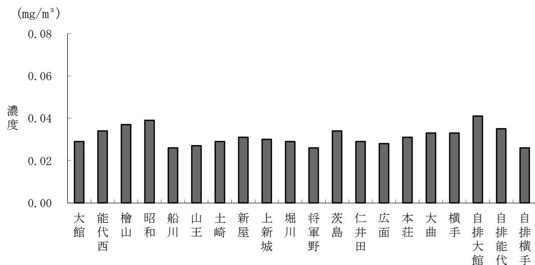
図24 浮遊粒子状物質の日平均値の年間 2%除外値 (平成28年度)
