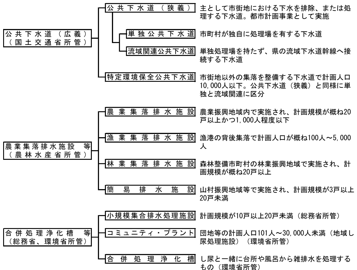
図 52 生活排水処理施設の種類
