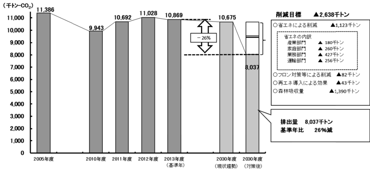
図 79 温室効果ガス排出量と削減目標
