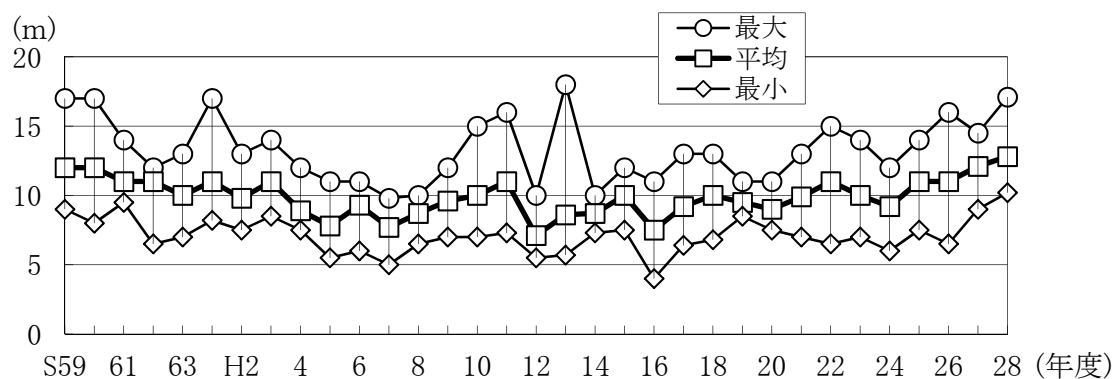
図44 十和田湖（湖心）の透明度の経年変化
