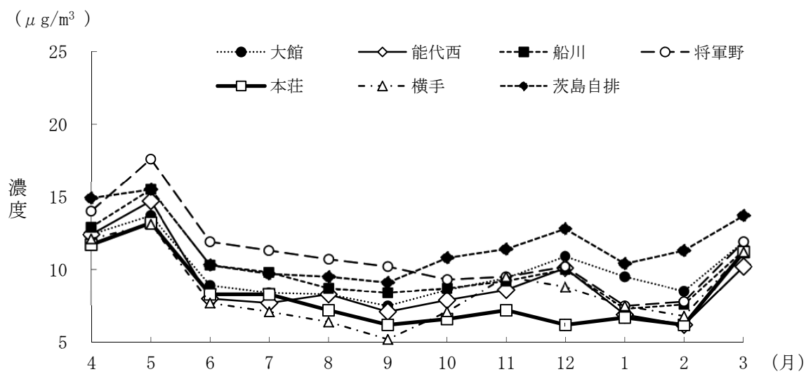
図28 微小粒子状物質の月平均値 (平成28年度)
