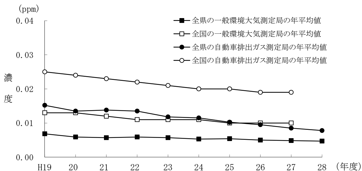
図19 二酸化窒素濃度の年平均値の経年変化
