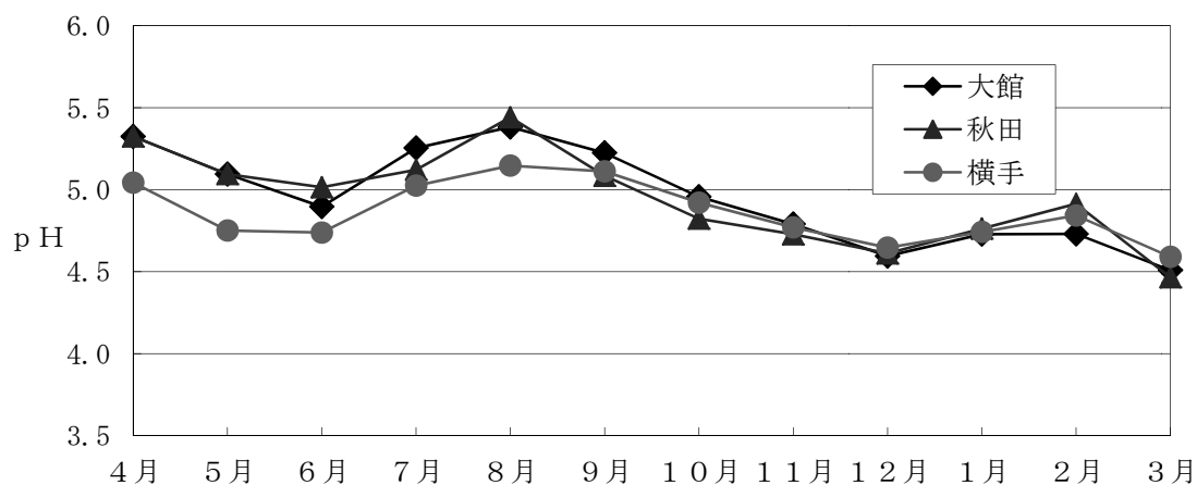
図 82 県内 3 地点における降雨・降雪の pH (月平均値) (平成 28 年度)
