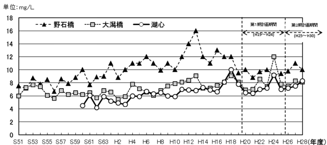
図 38 八郎湖の COD75% 値の経年変化
