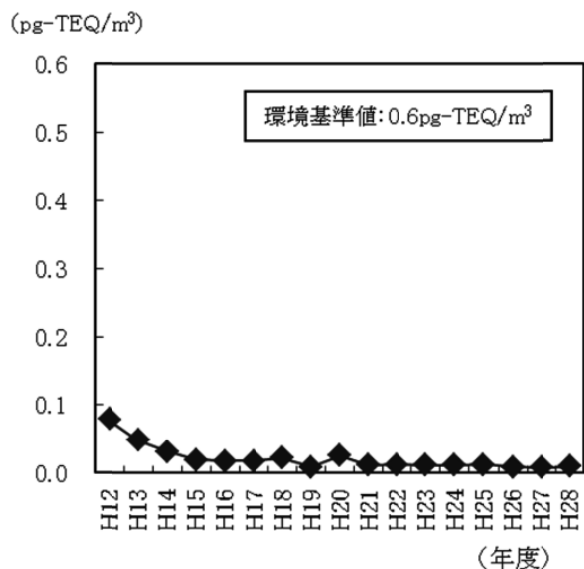
図 54 大気中濃度の経年変化（平均値）
