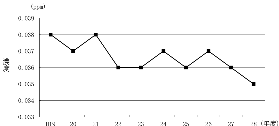
図22 光化学オキシダントの1時間値（昼間）の年平均値の経年変化（全県の大気測定局）
