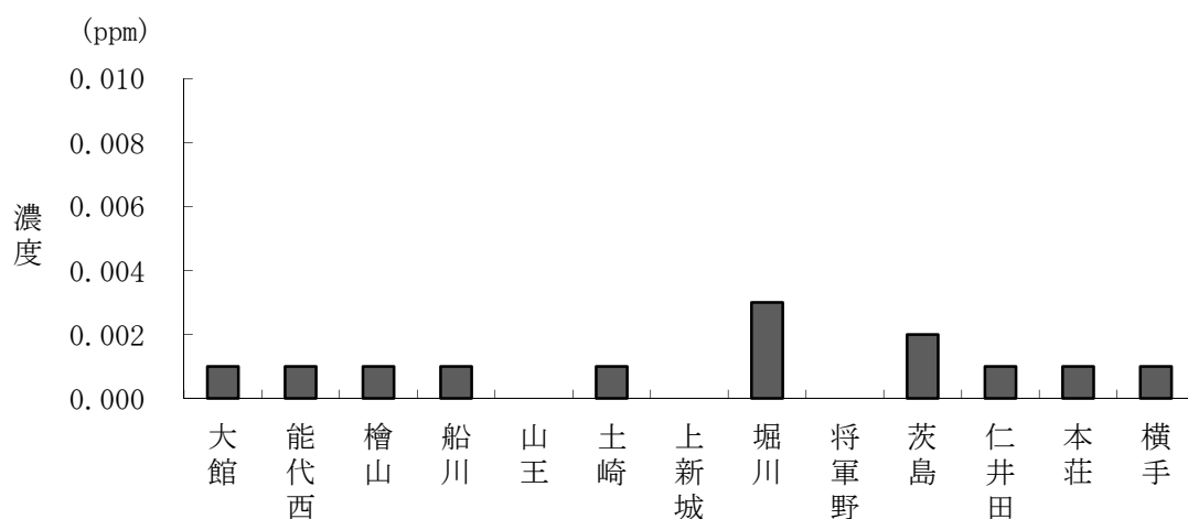
図14 二酸化硫黄の年平均値(平成28年度)
