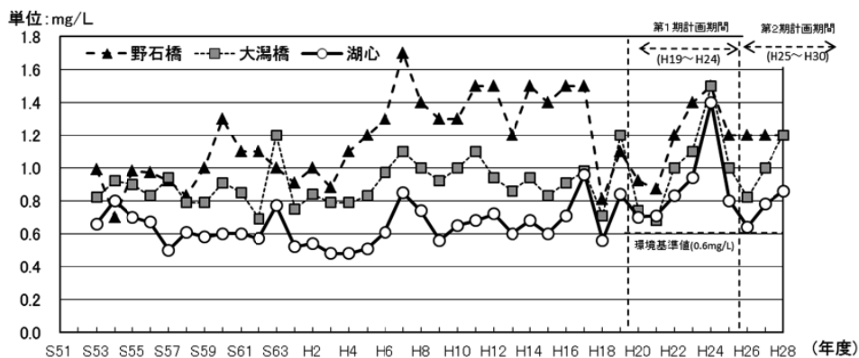
図 40 八郎湖の全窒素の経年変化（表層、年平均値）
