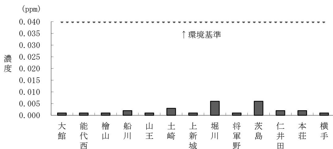
図15 二酸化硫黄の日平均値の年間2%除外値(平成28年度)
