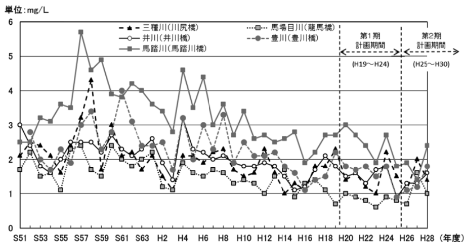
図 42 八郎湖流入河川の BOD75 値の変化
