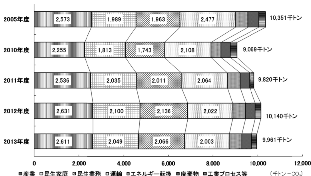
図 80 部門別二酸化炭素排出量の推移
