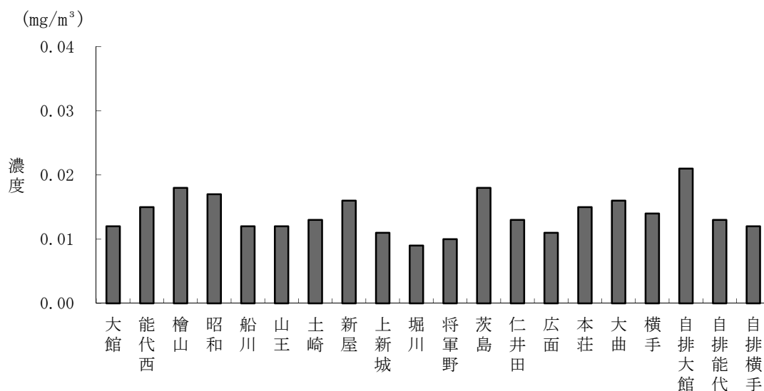
図23 浮遊粒子状物質の年平均値 (平成28年度)
