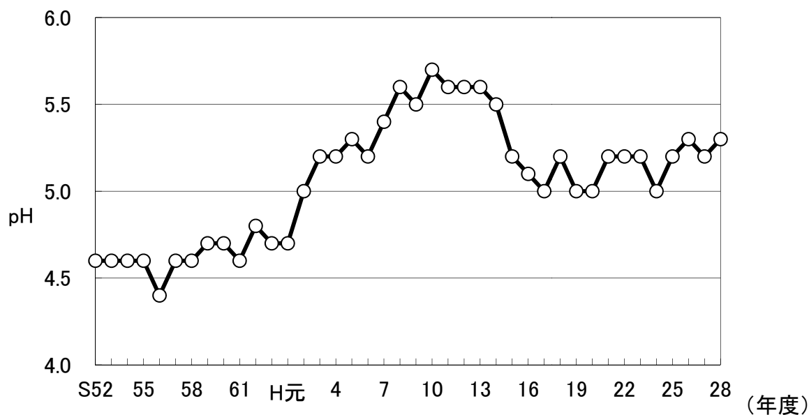
図 45 田沢湖 (湖心・0m・年平均値) の pH の経年変化
