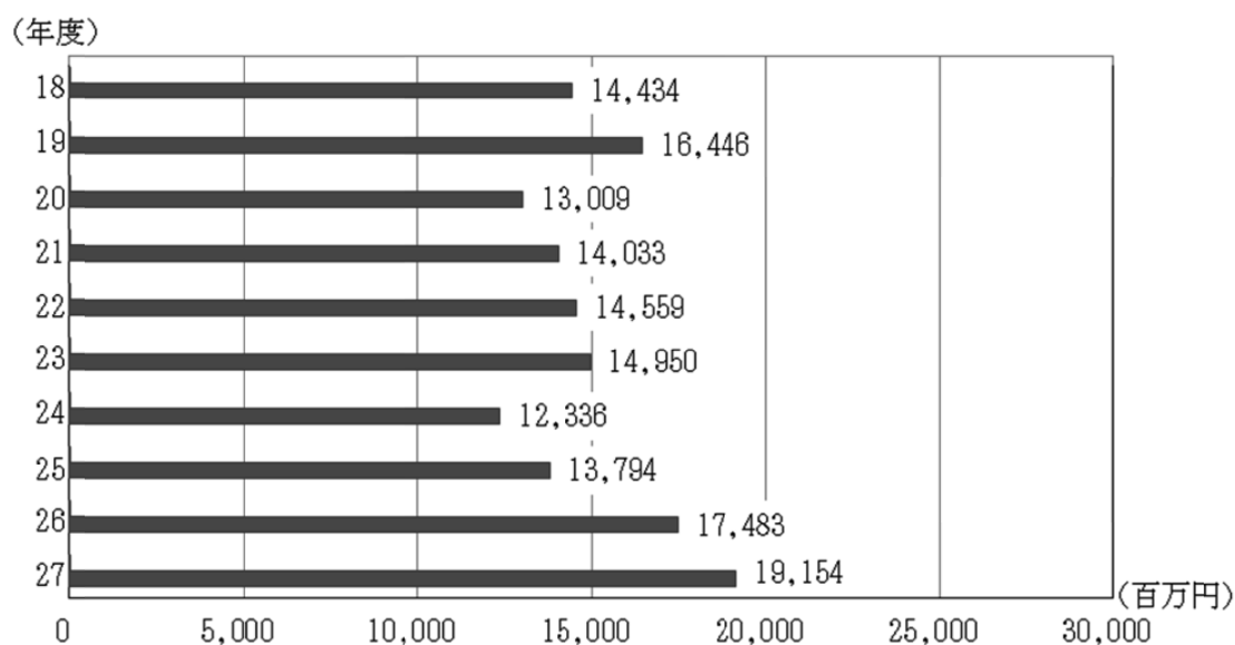
図 63 ごみ処理費用の推移
