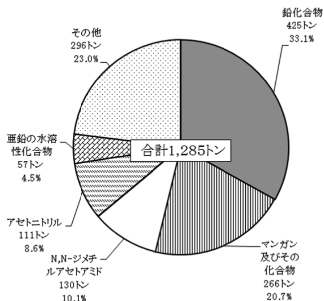
図 59 届出移動量の物質別内訳（平成 27 年度）
