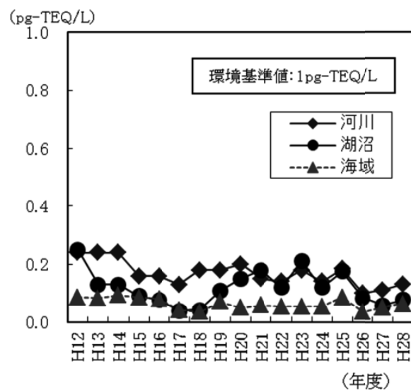
図 55 公共用水域水質中濃度の経年変化（平均値）
