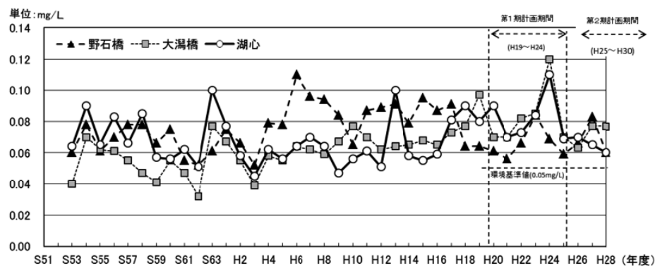
図 41 八郎湖の全りんの変化（表層、年平均値）
