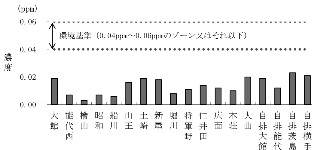
図18 二酸化窒素の日平均値の年間98%値（平成28年度）
