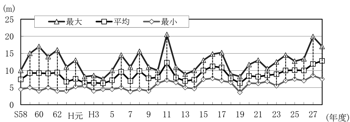
図 48 田沢湖（湖心）の透明度の経年変化
