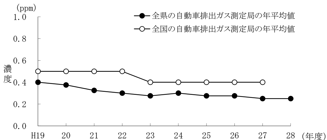
図20 一酸化炭素濃度の年平均値の経年変化
