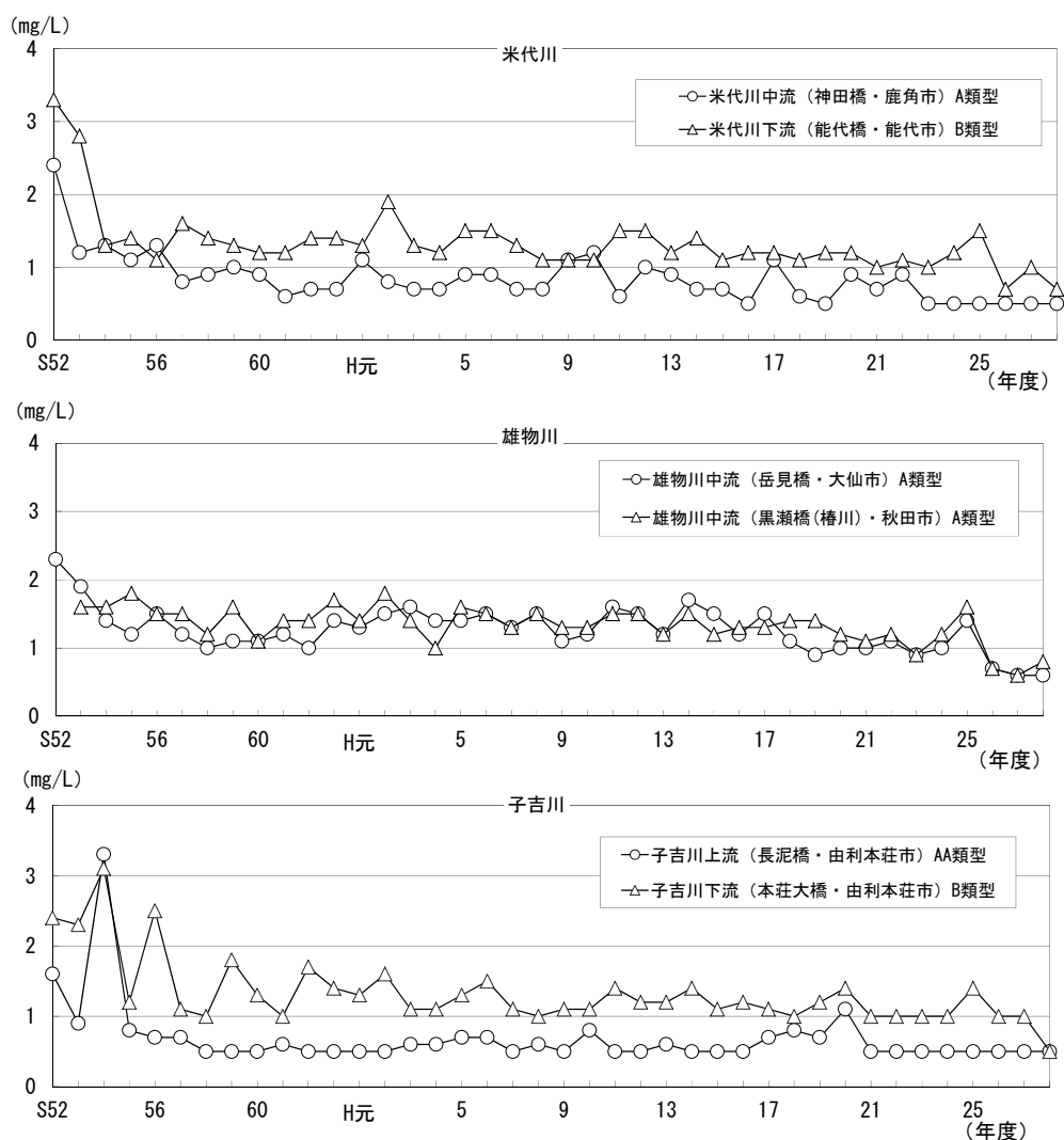
図 36 県内主要河川の BOD75%値の経年変化
