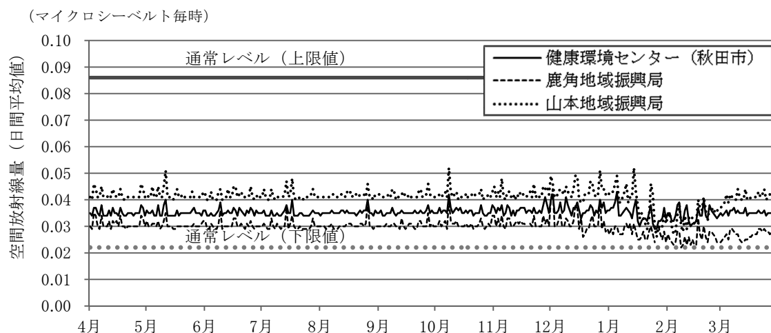
図 86 平成 28 年度の空間放射線量の推移（県中央から北部）
