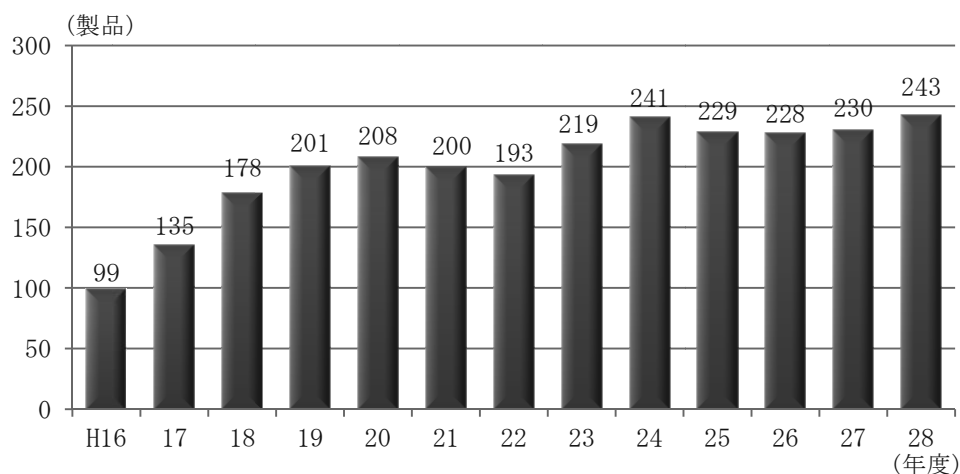
図76 認定製品数の推移
