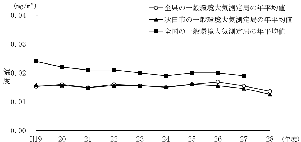
図25 浮遊粒子状物質濃度の年平均値の経年変化
