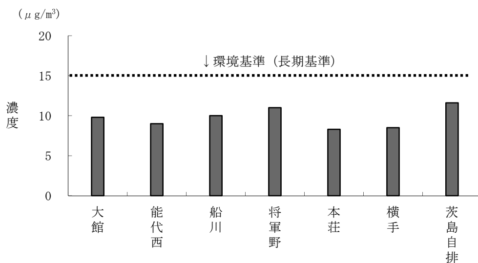
図 26 微小粒子状物質の年平均値（平成28年度）
