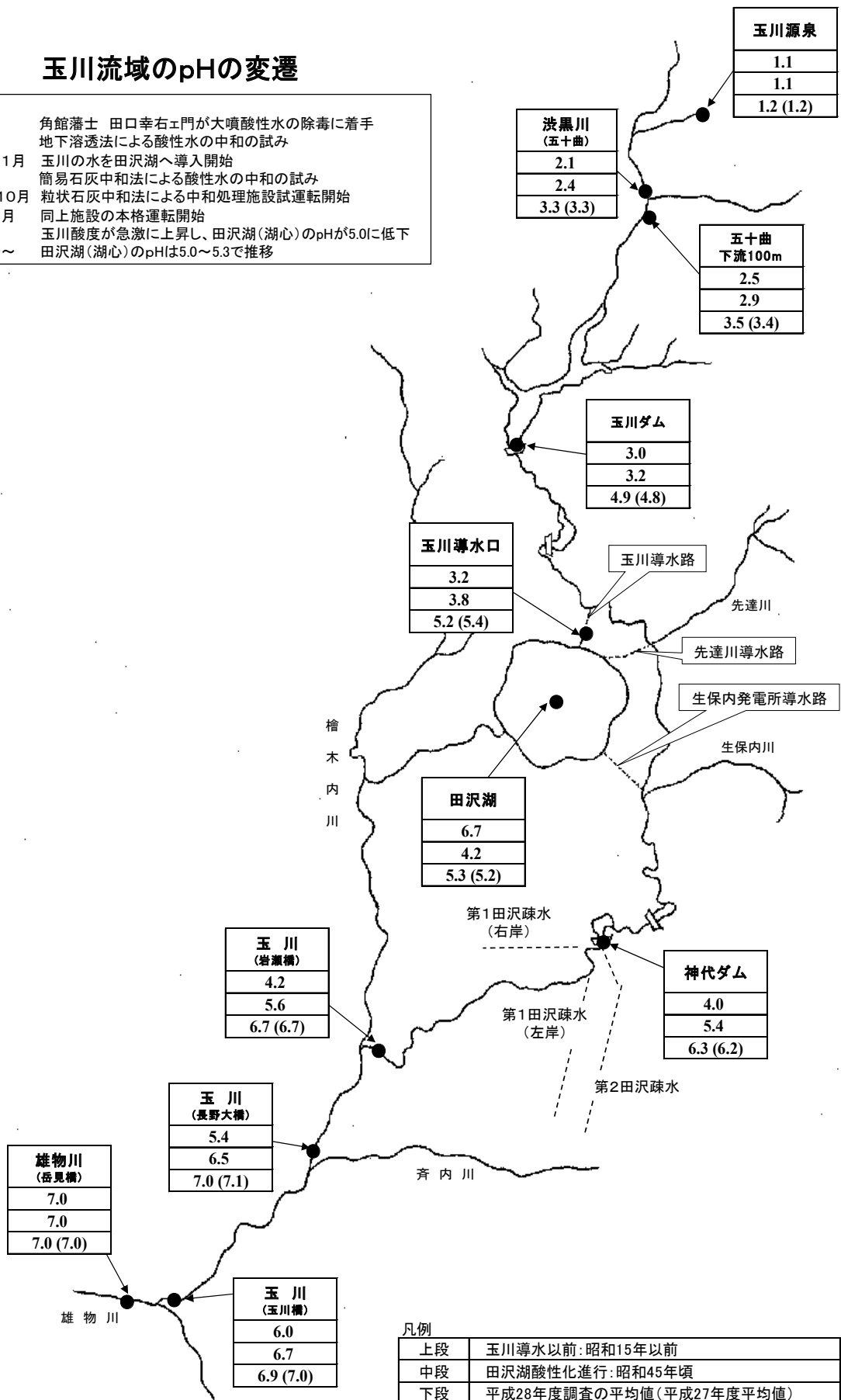
図 50 玉川流域の pH の変遷
