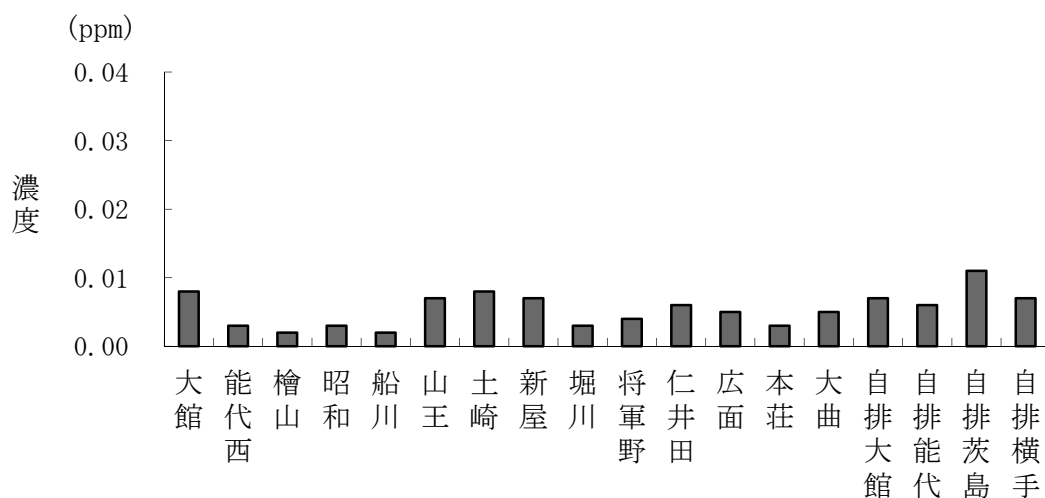
図17 二酸化窒素の年平均値（平成28年度）
