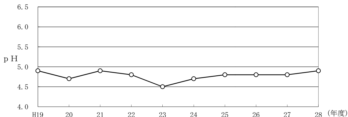
図 83 降雨・降雪の pH の経年変化 (全調査地点の平均値)
