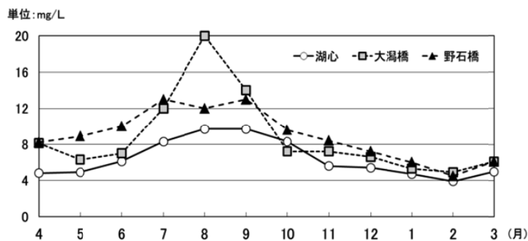
図 39 八郎湖の COD の経月変化（平成 28 年度）
