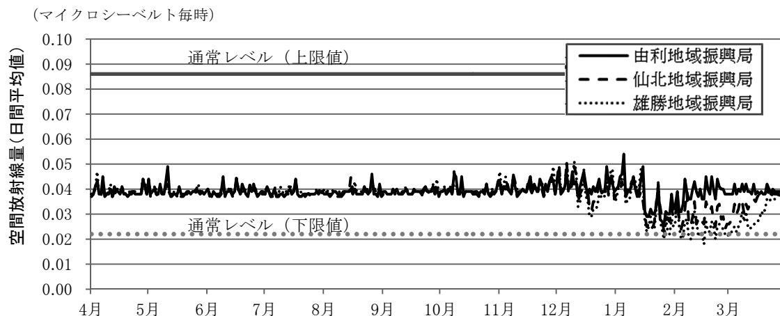
図 87 平成 28 年度の空間放射線量の推移（県南部）
