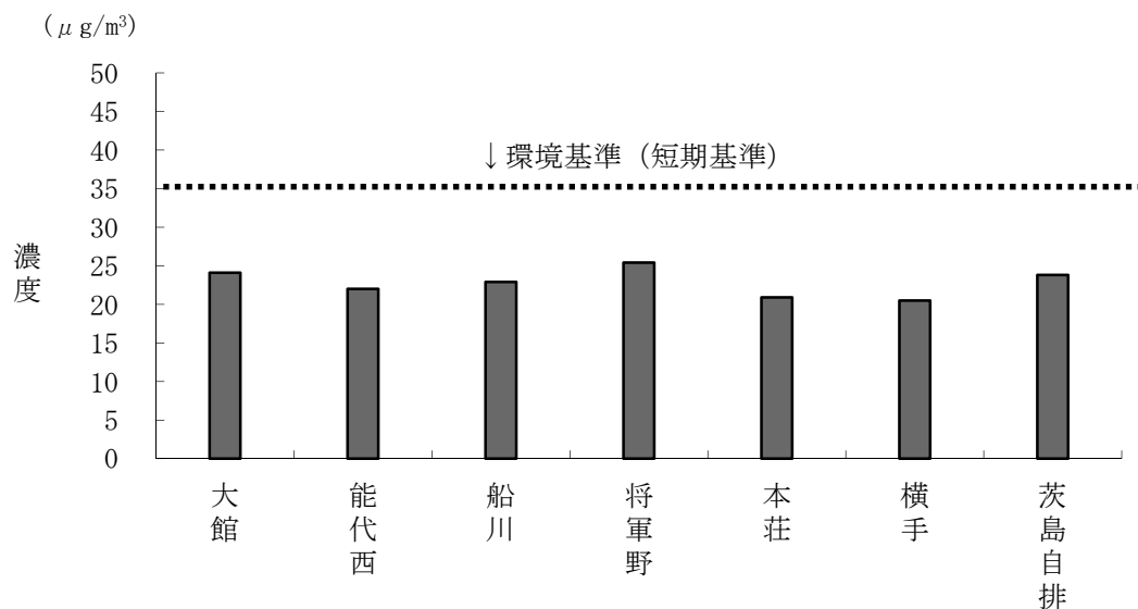
図27 微小粒子状物質の日平均値の年間98%値 (平成28年度)
