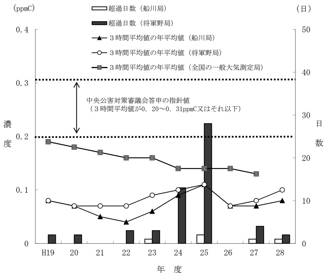
図29 非メタン炭化水素の3時間平均値及び指針値超可日数の経年変化
