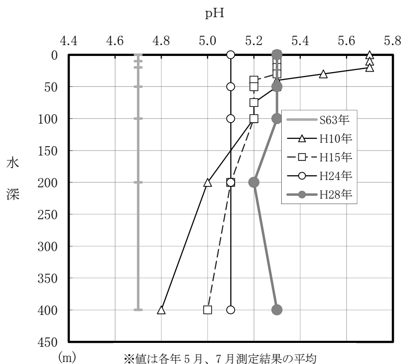
図 46 田沢湖（湖心・深度別）の pH 経年変化
