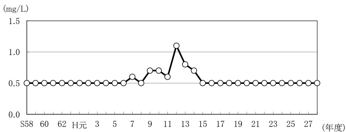
図 47 田沢湖（湖心）COD75%値の経年変化
