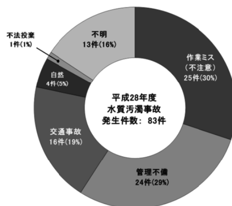
図 51 水質汚濁事故発生原因割合
