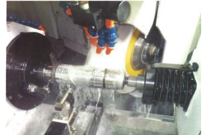
航空機部品の研磨工程
