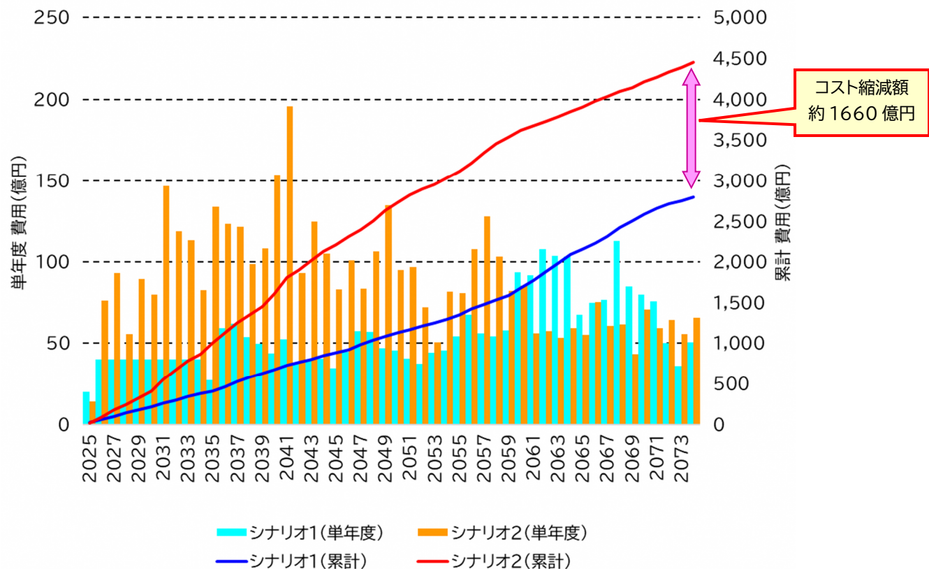
図 4.1 50年間の費用比較
