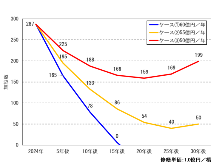
図 6.1 予算別における健全性Ⅲ橋梁数の推移予測 (年間 60 億円で健全性Ⅲが解消)
