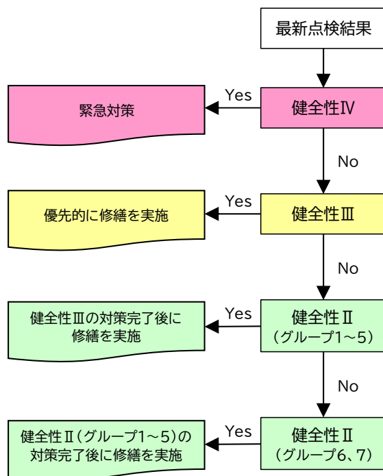
図 3.3 修繕計画の更新 イメージ
