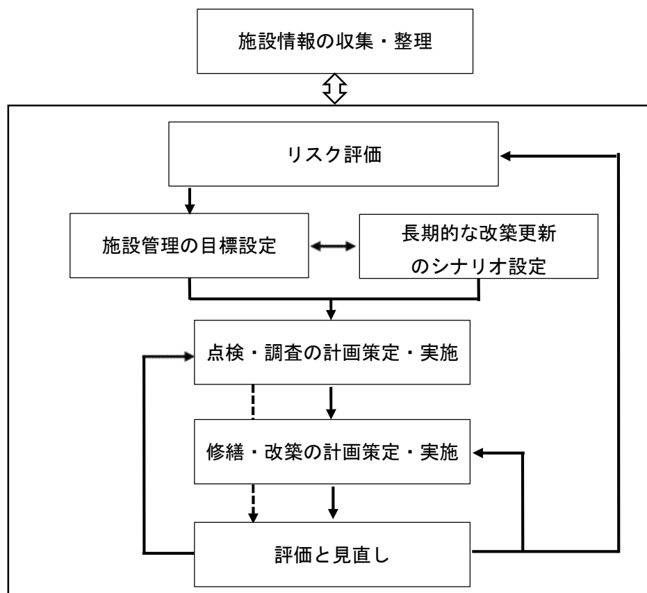
図3-I stockマネジメントの実施フロー
