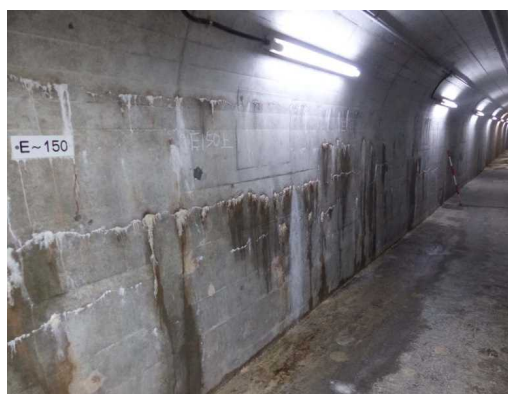
写 3-2- (2) 土木施設損傷例
