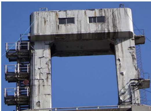
写 3-2-(1) 土木施設損傷例
