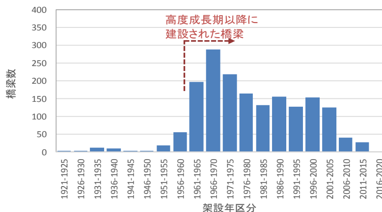
図 2.2 架設年別の橋梁数（橋梁 2m 以上 2,316 橋）
