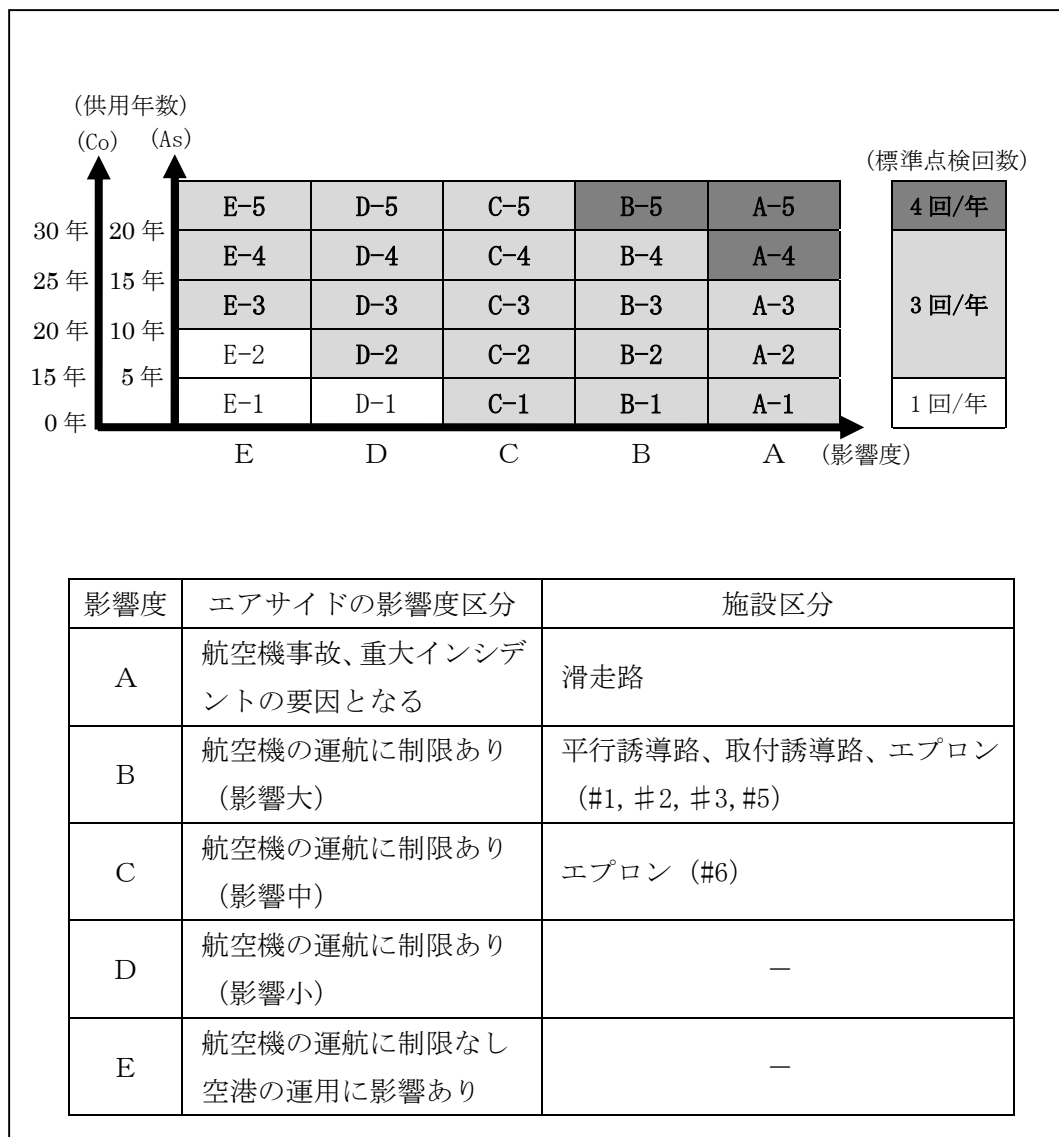
図一 1 滑走路等基本施設の巡回点検（巡回点検 I）の標準点検回数の設定方法
